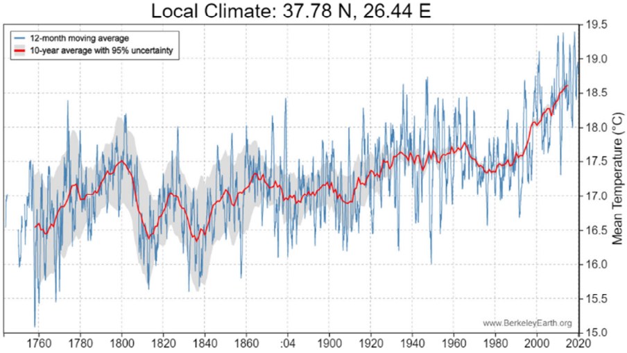
Resim 17: 1760-2020 yılları arası İzmir ve çevresinin iklim grafiği.
