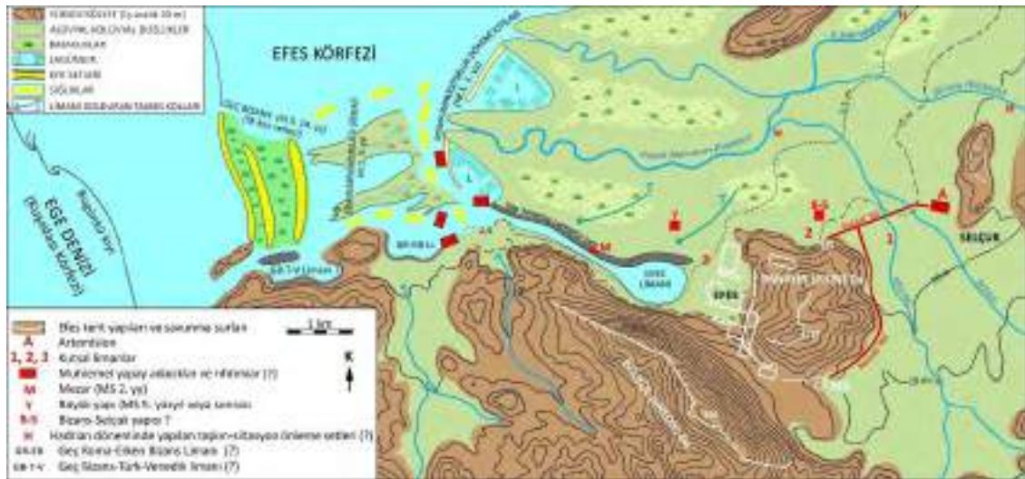
Şekil 13. Antik Efes'in Roma İmparatorluk ve Bizans dönemlerine ait paleocoğrafya haritası. Sürekli ilerleyen Küçük Menderes deltasının kıyı zonu “kuş ayağı” modelinde gösterilmiş olup, yerleri değişen ırmak yataklarının ve aralarında alçak bataklık alanların bulunduğu varsayılmıştır. Çatallanan ırmak yatakları (distributary channels) ağzındaki kumların dalga etkinliği ile karşılaşması sonucunda, geç Bizans döneminden günümüze kadar bataklıklar üzerinde kum sırtları (kıyı kumulları) oluşmuştur. Şekilden, erken Roma imparatorluğundan Büyük Liman'ın kullanımının sona erdiği geç Bizans dönemine kadar limanda sürekli dip taraması yapılmasının gerekli olduğu açıkça anlaşılmaktadır. Deltanın aşağı kesimindeki alüvyonlarda birkaç arkeolojik alanın bulunması, Leake (1835) tarafından Sperchios deltasının 1790-1830 yılları arasındaki aşağı kesimi için belirtildiği gibi, antik çağlarda burada muhtemelen yoğun bir tarımsal yerleşme olduğunu göstermektedir. Büyük Roma binaları, Lysimachus'un erken Helenistik zamanlardaki limanı üzerinde yapılmıştır. Öte yandan Kutsal Yol (Via Sacra), (bugünkü yüzeyin altında) Helenistik ve öncesindeki liman alanını kaplayan taşkın ovası sedimanları üzerinde uzanmaktadır. (ÇN: Şekil, içeriğine sadık kalınarak çeviren tarafından yeniden çizilmiştir).
