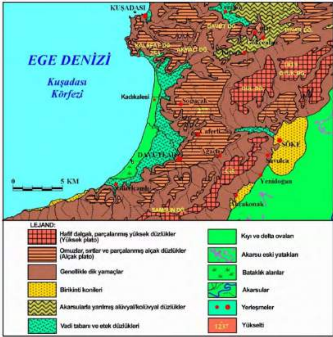
Şekil 4. Kuşadası-Davutlar kıyı düzlüğü ve çevresinin jeomorfoloji haritası.
