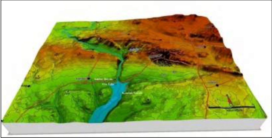
Şekil 3. Kocaköy Antiklinali ve Ambar Çayı Vadisi, Ambar Barajı etki alanı ve höyükleri gösteren blokdiyagram.
