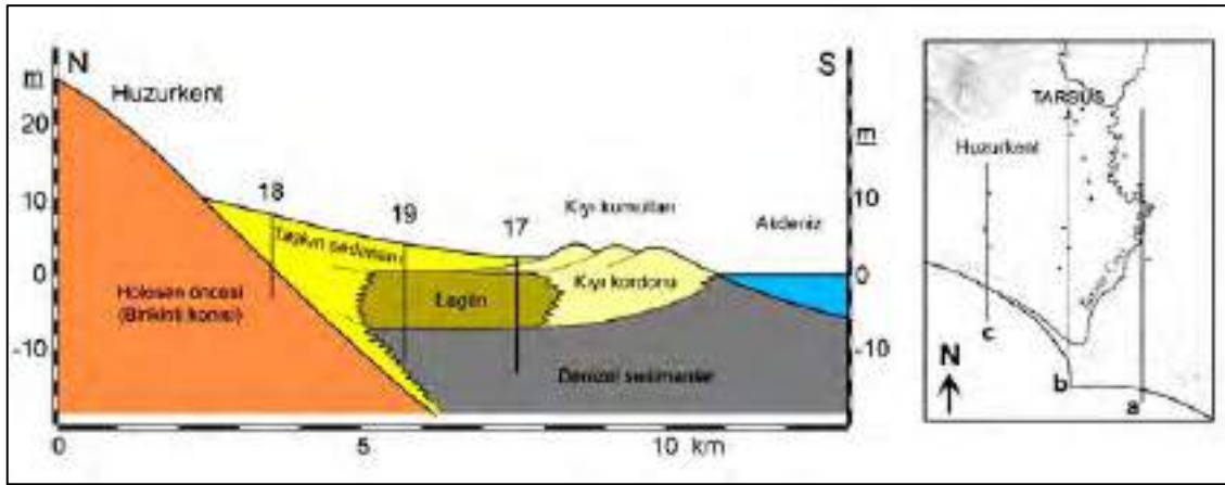
Şekil 10. Holosen öncesi birikinti konileri üzerindeki Tarsus ovasının (batı kesimi) alüvyal stratigrafisini gösteren kuzey-güney doğrultulu kesiti. Dikey çizgi ve numaraları sondajları göstermektedir. Küçük haritada “c” harfi kesit yer ve doğrultusunu gösterir.
