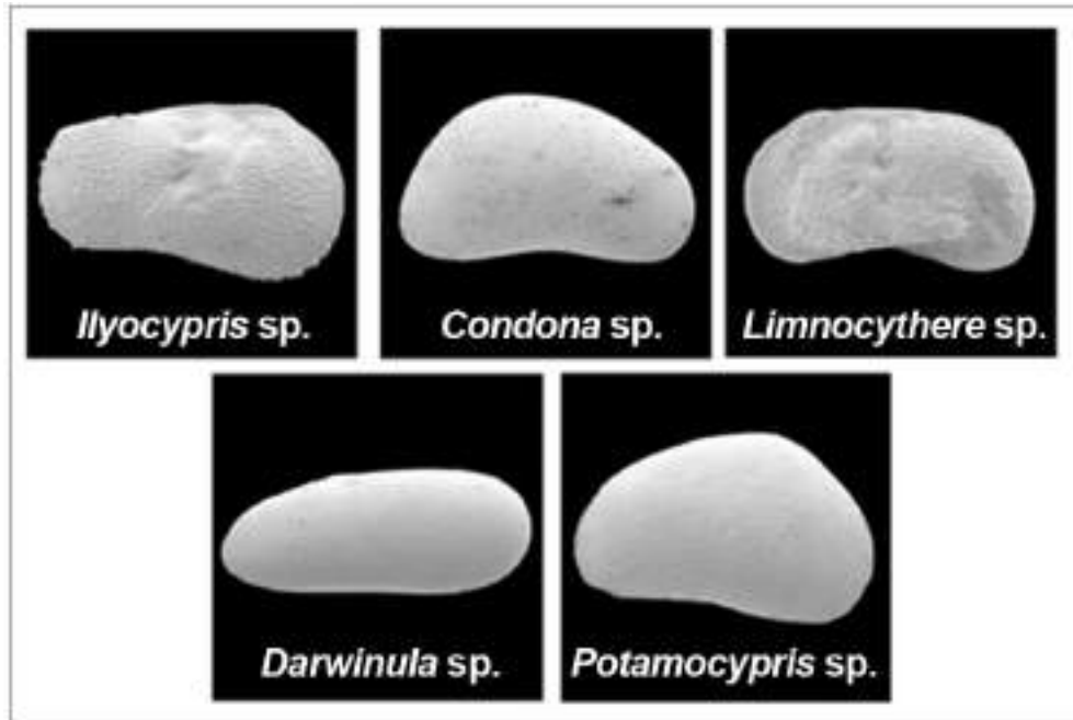
Şekil 9. Madra Çayı Deltası (Altınova) AO-12 sondajında çok sayıda tespit edilen tatlı su Ostracodları (SEM, Gökçen, 1997).
