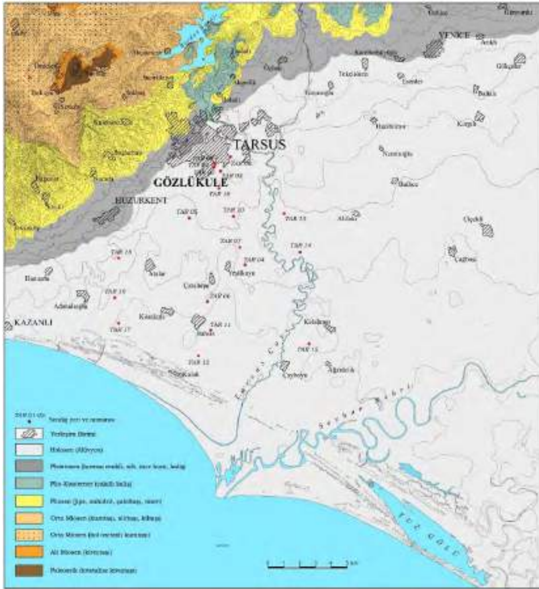
Şekil 7. Tarsus ve Gözlükule Höyüğü çevresinin jeoloji haritası.
