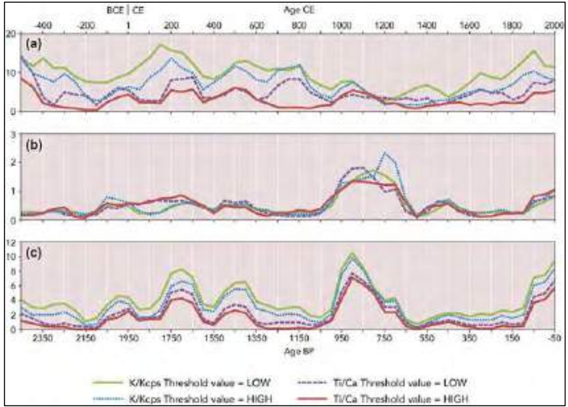
Şekil 6. (a) Kırıntılı tabaka frekansı, (b) tek kırıntılı tabaka kalınlığı ve (c) NAR10 karot dizisinde 2500 cal BP'den beri 50 yıllık toplam kırıntılı tabaka kalınlığı (BCE: Milattan Önce, CE: Milattan Sonra).
