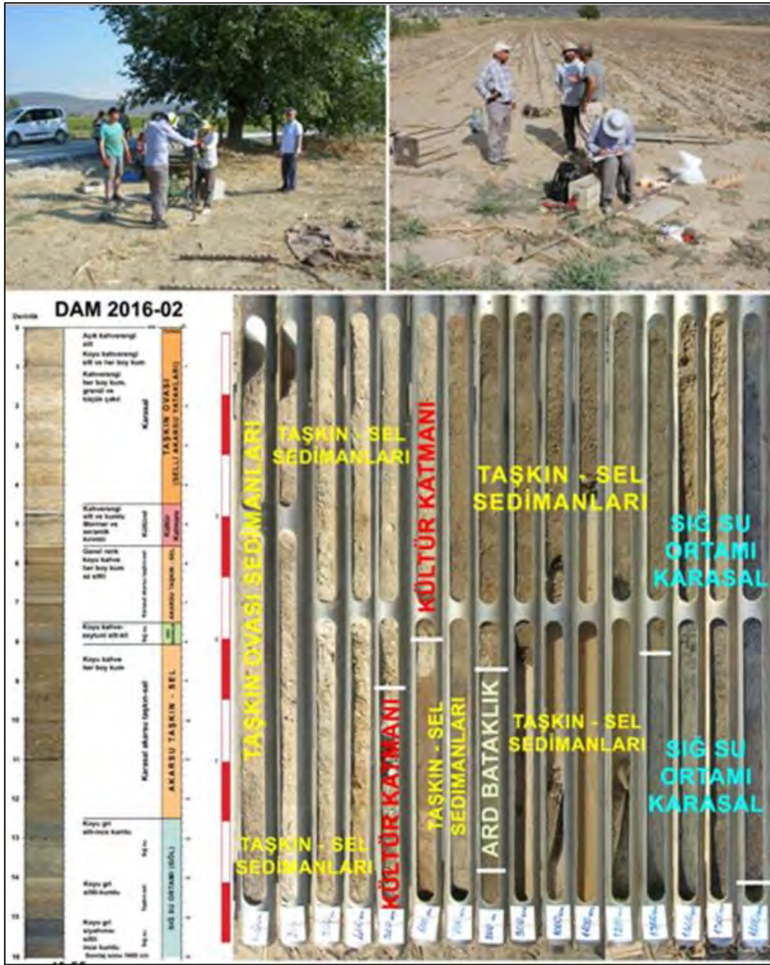
Şekil 10. Damlıboğaz önlerindeki ovada yapılan ve 16 metre derinliğe inilen DAM-2016-02 numaralı sondaj çalışmasından görüntüler, sondaj logu-karotu ve ortam özellikleri (Vardar vd., 2017).
