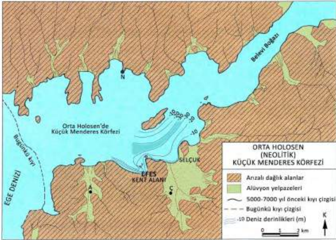
Şekil 4. Holosen transgresyonunda denizin en fazla sokulduğu Orta Holosen'e (~6000 yıl B.P.) ait Küçük Menderes (Efes) Körfezi haritası. Bu zamana ait iki arkeolojik alan bilinmektedir: Bunlar kuzeyde, Kuaterner alüvyonlarından oluşan bir etek sırtı üzerindeki Neolitik alan (N) ile Efes antik kentinin Magnesian kapısının yaklaşık 400 m güneydoğusundaki Çukuriçi (Ç) höyüğüdür (muhtemelen Kalkolitik) (A: Sonraki çalışmalarla batıdaki antik Kenchios (Arvalya) vadisinde bulunan Arvalya höyüğü. ÇN 2). Kuzeydeki alan, denizin hemen kenarındadır ve burada yiyecek artığı denizel kavkılar ile çanak-çömlek kırıkları bulunmaktadır. Güneydeki Çukuriçi höyüğü ise denizin küçük bir girintisinin gerisinde, o zamanki kıyıdan 1,5 km kadar içeride, alüvyal vadi tabanında bulunmaktadır. Güney kıyı çizgisi ile körfez ortasındaki mermer yapılı ada-horst (Kurudağ, antik Syrie) arasında su derinliği çizgileri gösterilmiştir.
