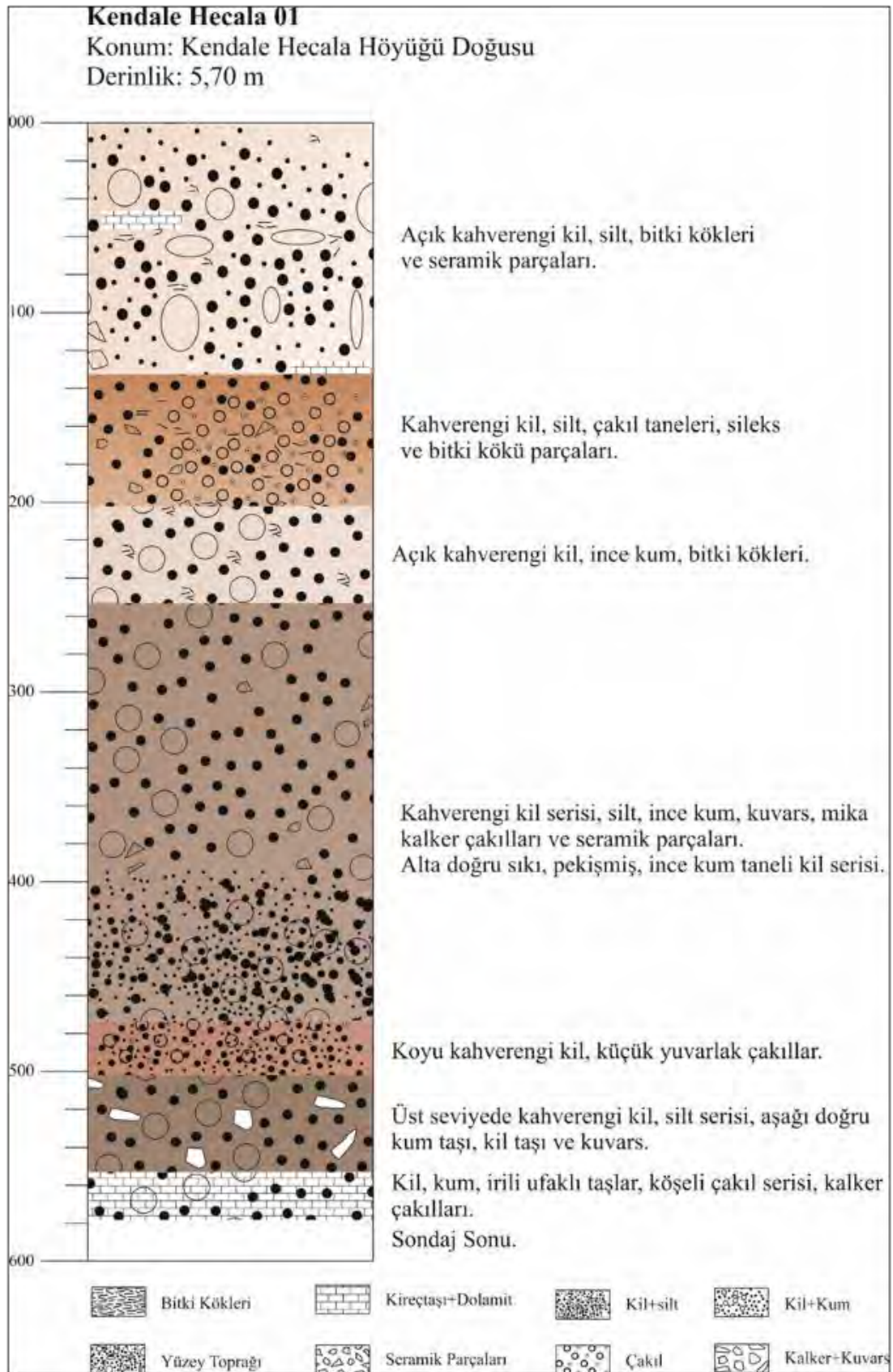
Şekil 7. Kendale Hecala 1 nolu sondaj litoloji loğu.
