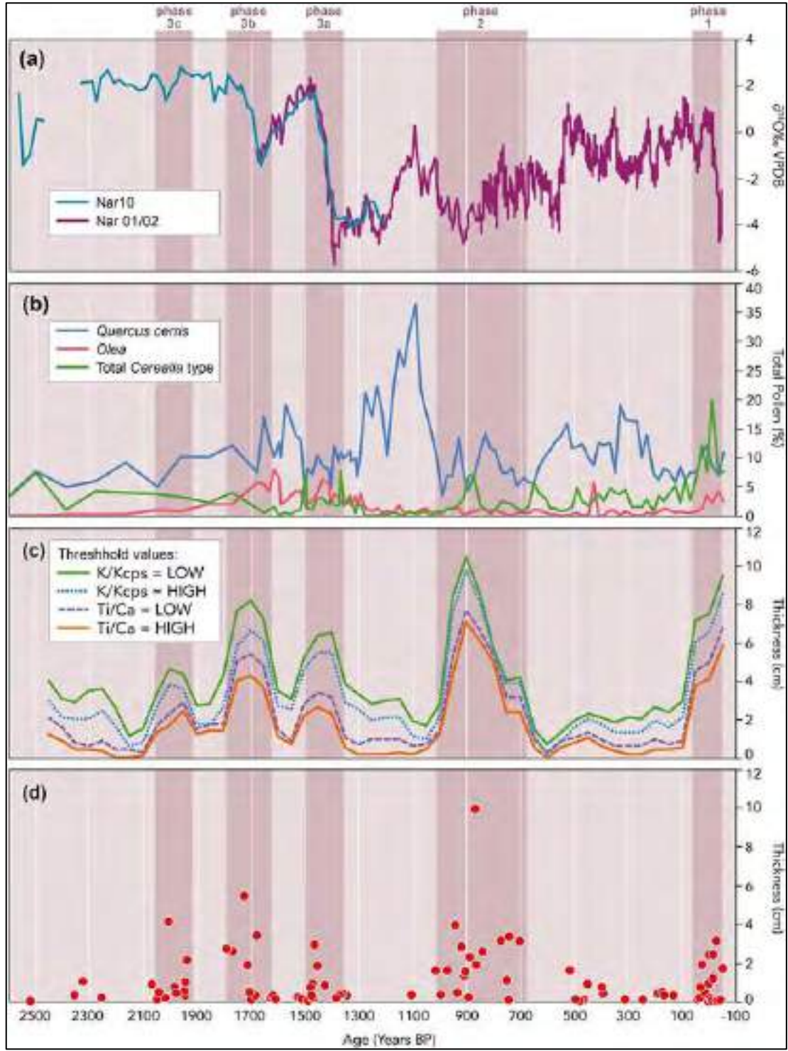
Şekil 7. NAR10 karotundakidaki kırıntılı katmanlar ile iklim ( \delta\text{O}^{18} ) ve arazi örtüsü değişimi (polen) grafikleri (kararlı izotop verileri; Jones ve diğ. (2006), Dean ve diğ. (2015b); polen verileri kısmen England ve diğ. (2008). Koyu renkli şeritler, Nar Gölü'ne gelen sediment taşınımının ana dönemlerini göstermektedir.
