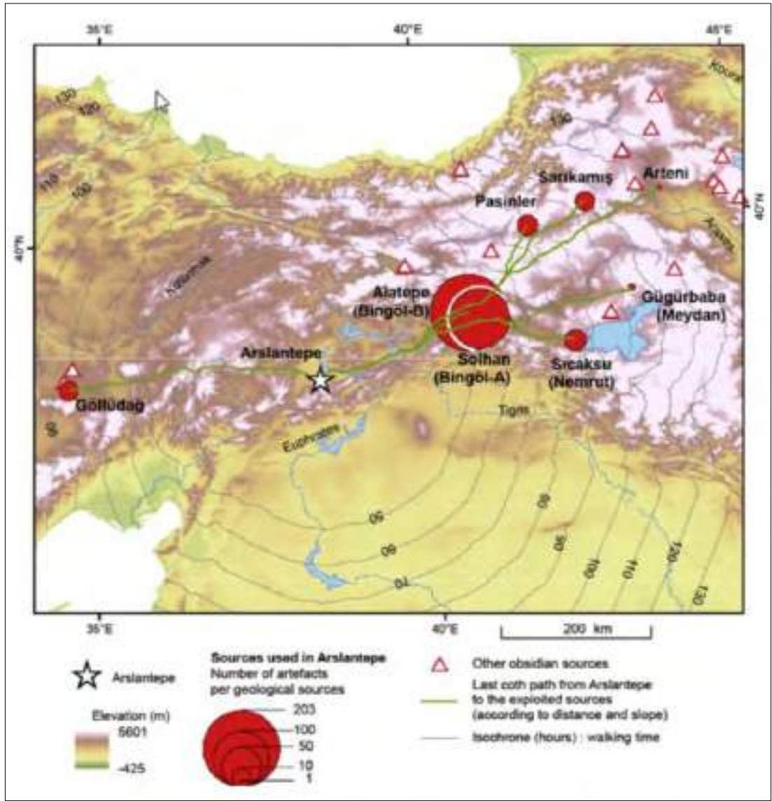
Şekil 7. Arslantepe Höyüğü Geç Kalkolitik- Erken Tunç Çağı popülasyonlarına tarafından kullanılan obsidiyenlerin kaynak alanları (Kaynak: Mouralis vd., 2018).
