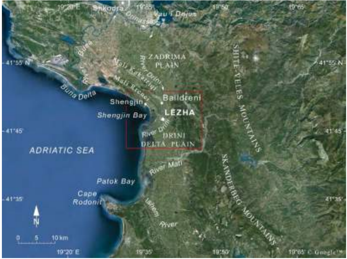
Şekil 1. Kuzey Arnavutluk'un uydu görüntüsü.
