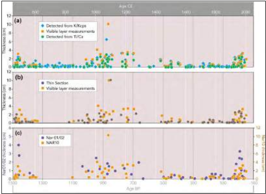
Şekil 3. Son 1500 yıllık kırıntılı tabaka kalınlığı ve yaşı; (a) Itrax tarama ve görsel kayıtlı ölçümü karşılaştıran NAR10 karotları; (b) görsel ve ince kesit ölçümlerinin karşılaştırılması, (c) NAR10 ve NAR01/02 karotları için görsel ölçümler (dikey ölçekteki fark dikkat edin). MS 1950’den önceki yıllarda zaman ölçeği.
