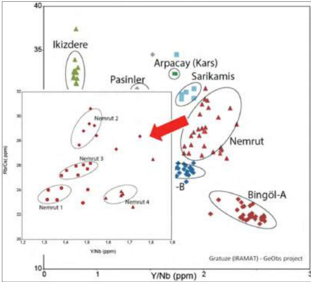
Şekil 4. Nemrut Obsidiyenlerinin Jeomkimyasal analiz sonuçları (Kaynak: Akköprü vd., 2017).
