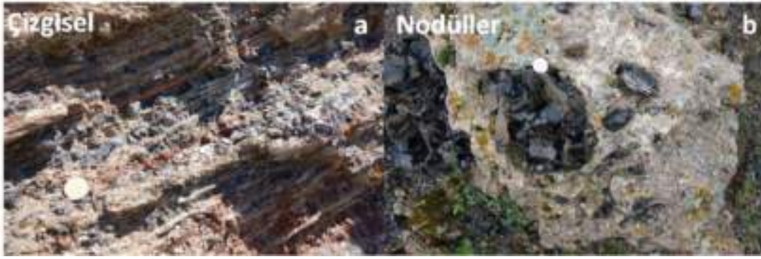
Şekil 3a-b. Nodüler ve çizgisel formdaki Nemrut Volkanı obsidiyenler (Kaynak: Akköprü vd., 2017).
