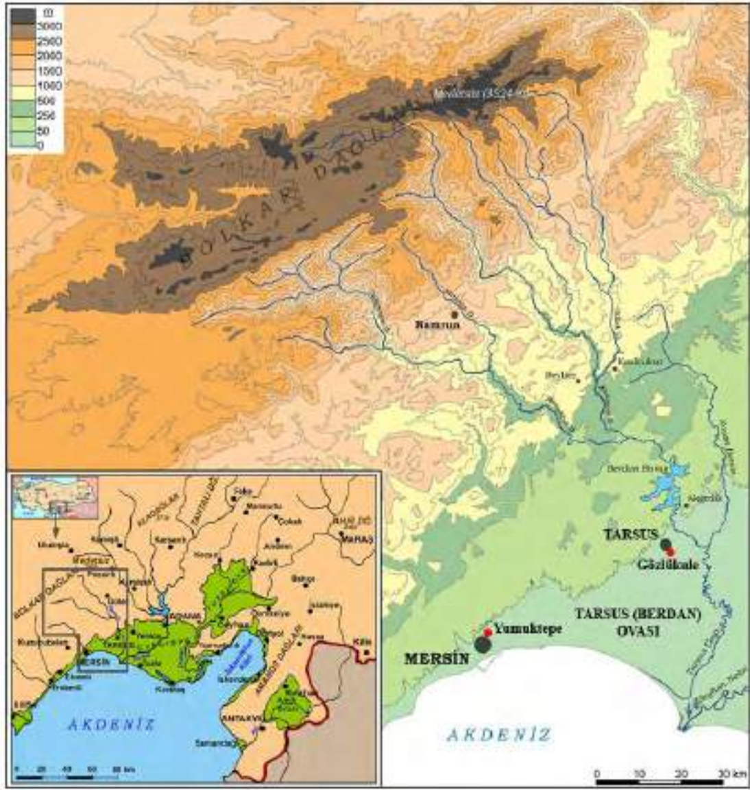
Şekil 3. Tarsus çayı havzasının topoğrafik ve oro-hidroğrafik haritası ve Tarsus ovasının lokasyonu.
