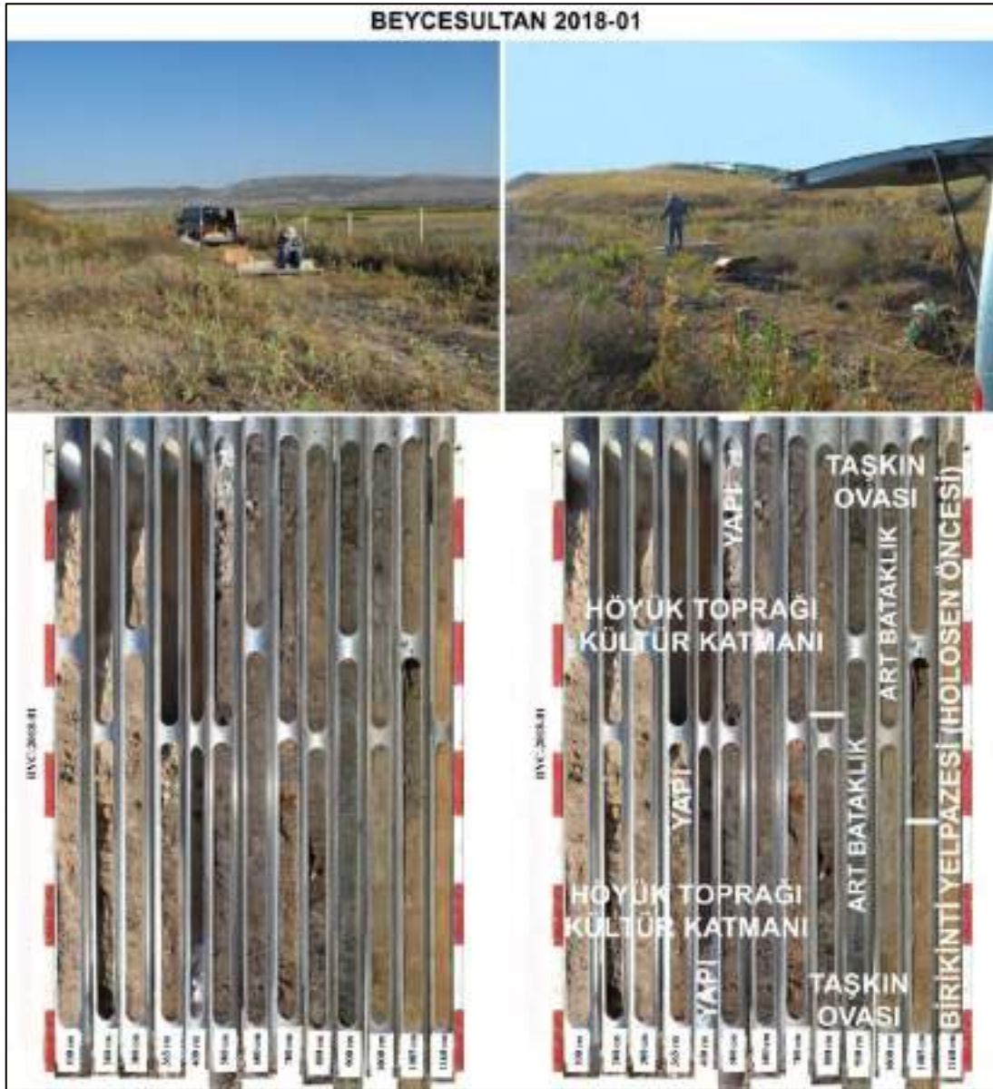
Foto 2. Beycesultan Höyüğü kuzey eteğinde yapılan BYC 2018-01 numaralı sondaja ait sedimanlar ve yansıttıkları ortamlar.
