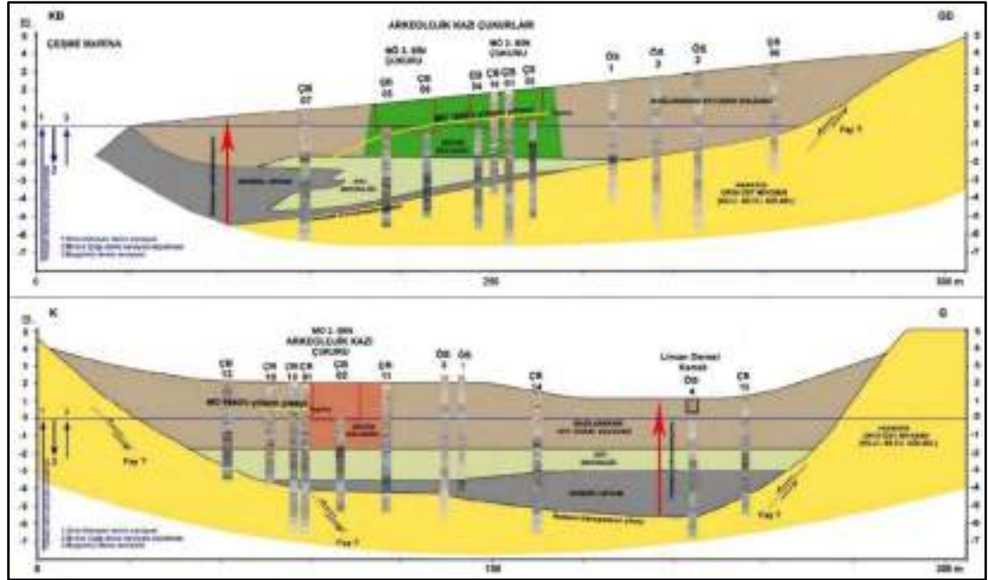
Şekil 27. Bağlararası kıyı ovası alüvyal-kolüvyal dolgularının KB-GD (üstte) ve K-G doğrultulu kesiti (Altta) (Vardar vd., 2017; Vardar ve Öner, 2017a; Vardar ve Öner 2017b; Öner vd., 2019).
