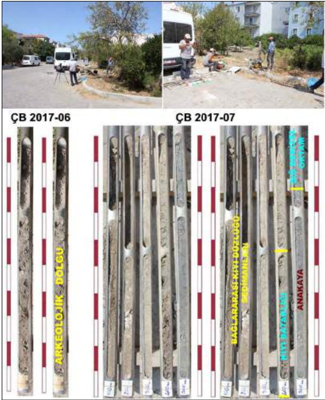
Şekil 20. ÇB-2017-06 ve ÇB 2017-07 numaralı sondaj çalışmalarından çalışmasından görüntüler, sondaj logu ve ortam özellikleri.
