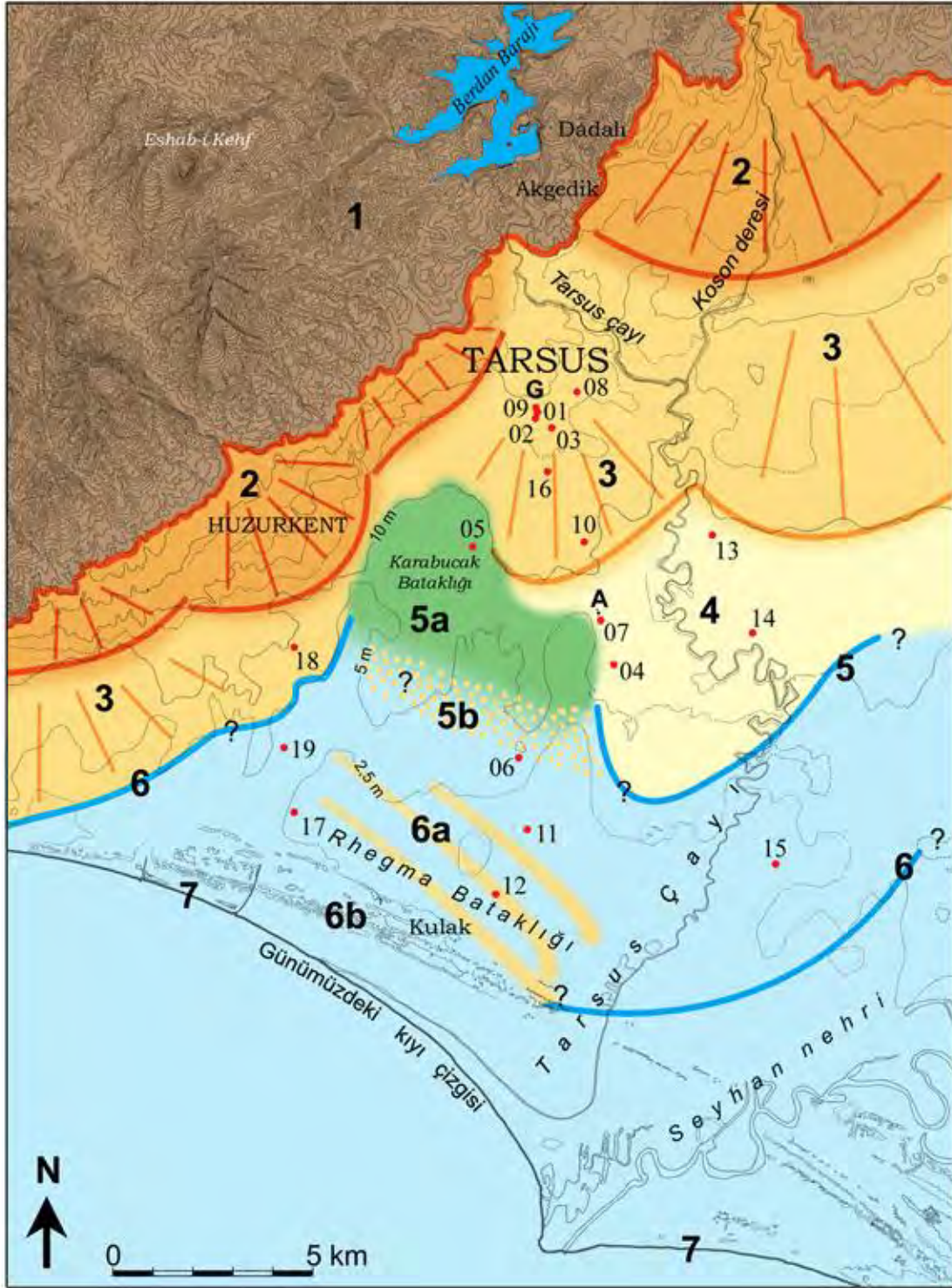
Şekil 13. Tarsus ovasının paleocoğrafya haritası. 1) Engembeli dağlık alan. 2 ve 3) Eski (Holosen öncesi) birikinti konileri. 4) Tarsus çayının Erken Holosen delta-taşkın ovası. 5) Orta Holosen kıyı çizgisi (Holosen transgresyonunun ulaştığı maksimum kıyı çizgisi). 5a) Orta Holosen kıyı bataklığı ya da kısmen lagün ortamı. 5b) Orta Holosen kıyı ortamının kıyı kordonları ya da kıyı dilleri boyunca uzanan geçiş formasyonları. 6) Tarsus çayının Orta-Geç Holosen delta kıyısı ve; 6a) kıyı kordonu ve kıyı kumulları (kısmen güncel kumullar). 6b) güncel kıyı kordonu ve kıyı kumulları. 7) Günümüz kıyı çizgisi. G: Gözlükule höyüğü. A: Aliefendioğlu höyüğü. Kırmızı noktalar sondaj yerlerini göstermektedir. İzohipsler 10 m aralıklarla (yalnızca ova alanında 5 ve 2,5 metre) çizilmiştir.
