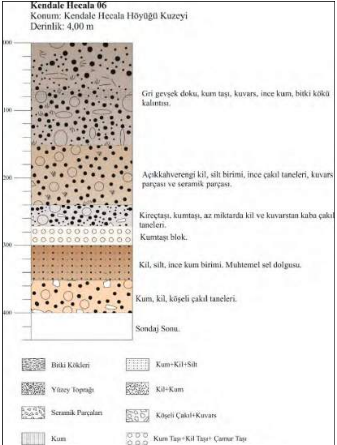
Şekil 12. Kendale Hecala 6 nolu sondaj litoloji loğu.
