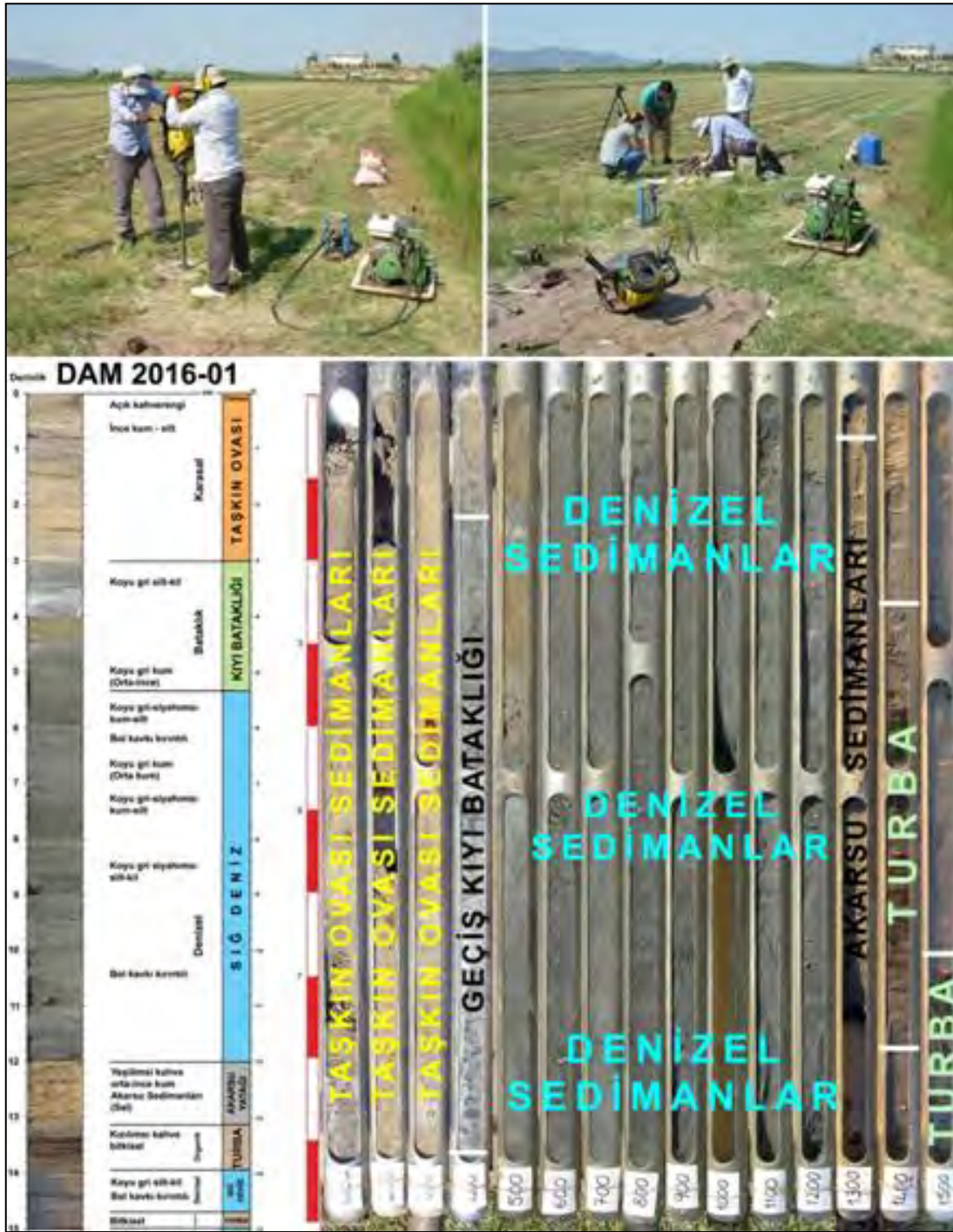
Şekil 8. Güllük körfezi kıyıları ile Pilav Tepe arasında yapılan ve 15 metre derinliğe inilen DAM-2016-01 numaralı sondaj çalışmasından görüntüler, sondaj logu-karotu ve ortam özellikleri (Vardar vd., 2017).
