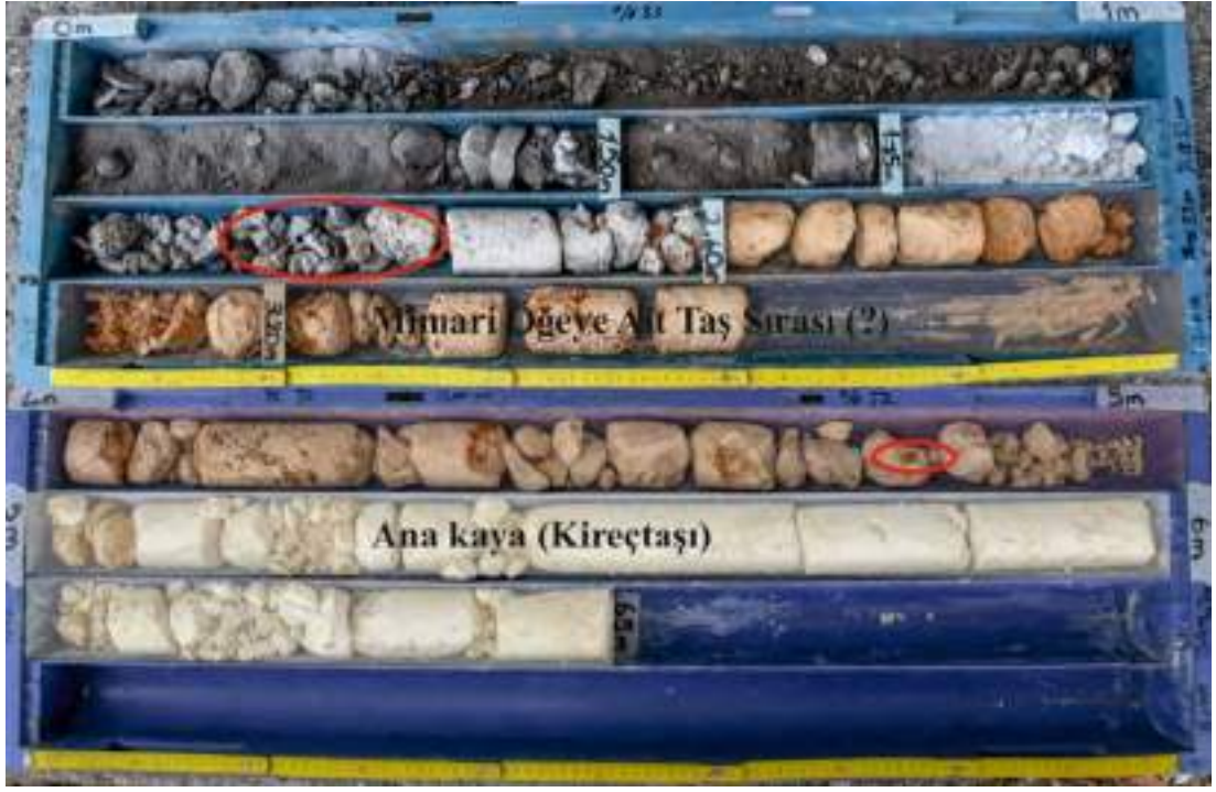
Foto 5. Ambar Höyük 1 nolu sondajın karot örnekleri (Karot uzunluğu 1m).
