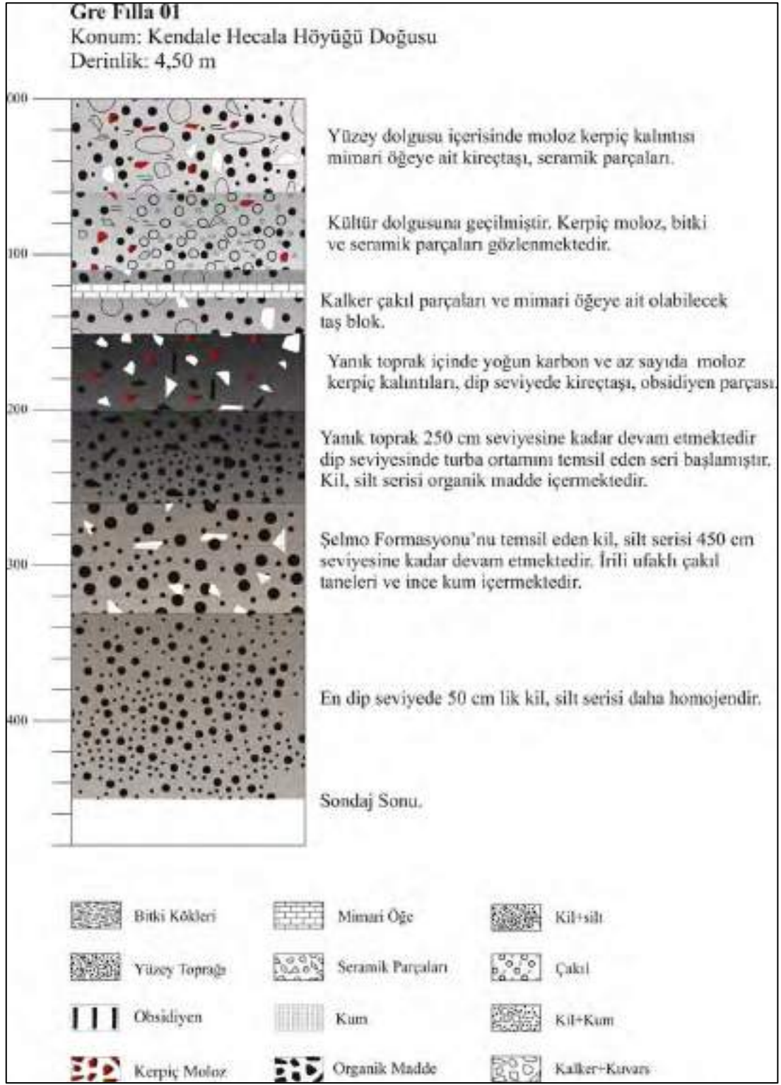
Şekil 6. Gre Filla Höyük nolu sondajı litoloji loğu.
