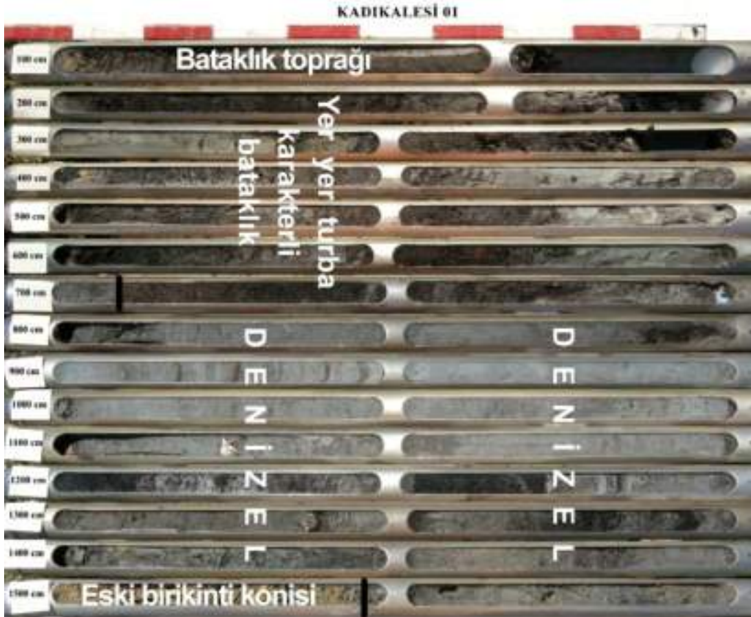
Şekil 15. Kadikalesi-01 sondajına ait sedimanların ortam özellikleri.
