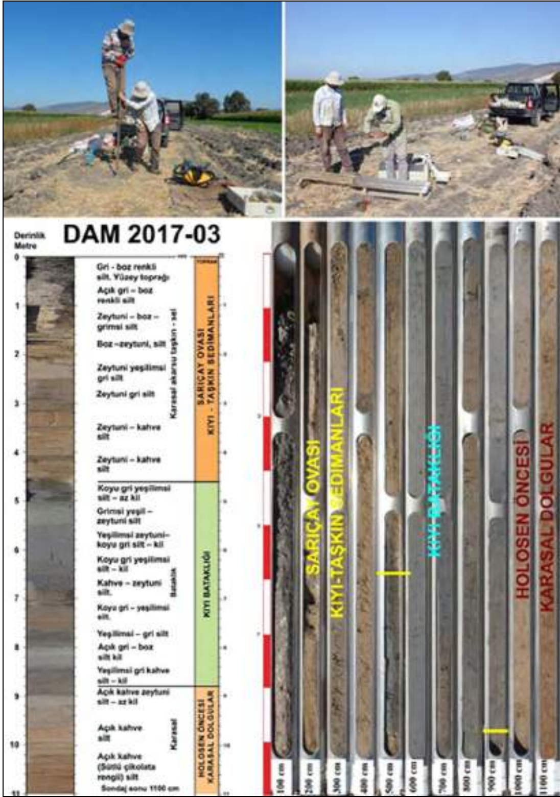
Şekil 17. Pilav Tepe kuzeybatı eteklerine yakın yapılan ve 11 metre derinliğe inilen DAM-2017-03 numaralı sondaj çalışmasından görüntüler, sondaj logu-karotu ve ortam özellikleri.
