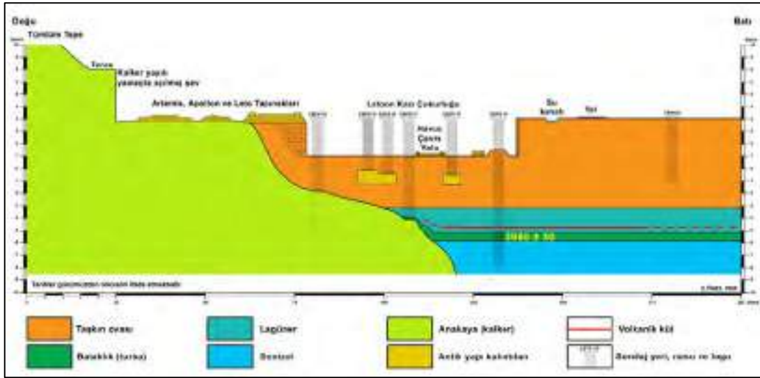
Şekil 16. Letoon kazı alanı ve çevresindeki sondajlara göre hazırlanan D-B yönlü kesit.
