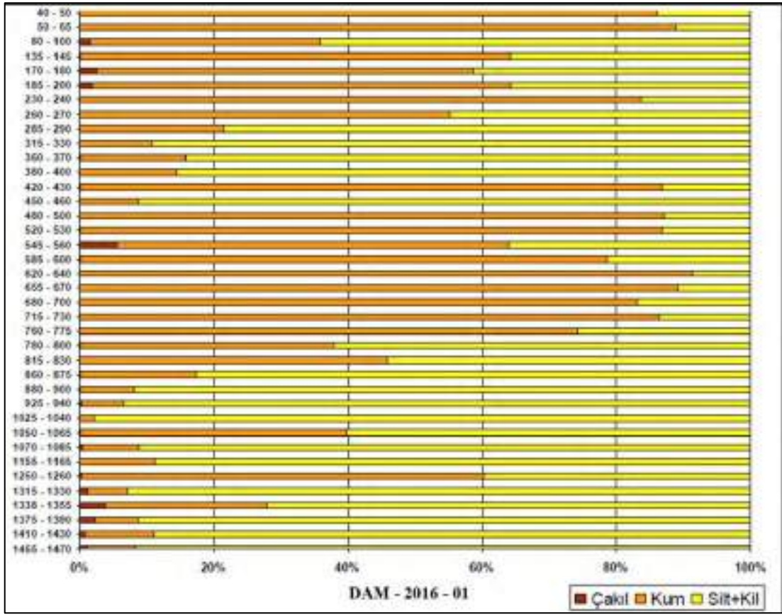
Şekil 7. Damlıboğaz ovasında gerçekleştirilen DAM-2016-01 Nolu sondajın tane boyu dağılımı.
