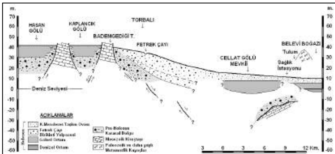
Şekil 3. Torbalı Ovası alüvyal dolgularının kesiti (Vardar ve Sarıöz, 2006).
