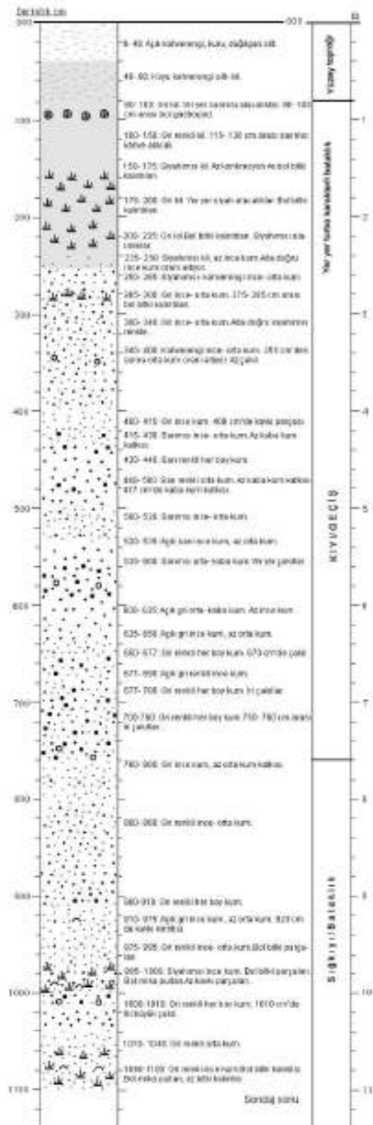
Şekil 23. Kadıkalesi-10 nolu sondaj logu.
