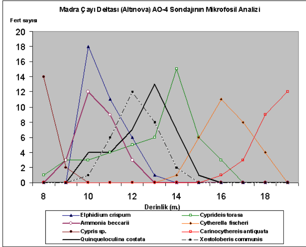
Şekil 4. AO-04 sondajının denizel sedimanlarından alınan Foraminifer ve Ostracodların dağılışı.
