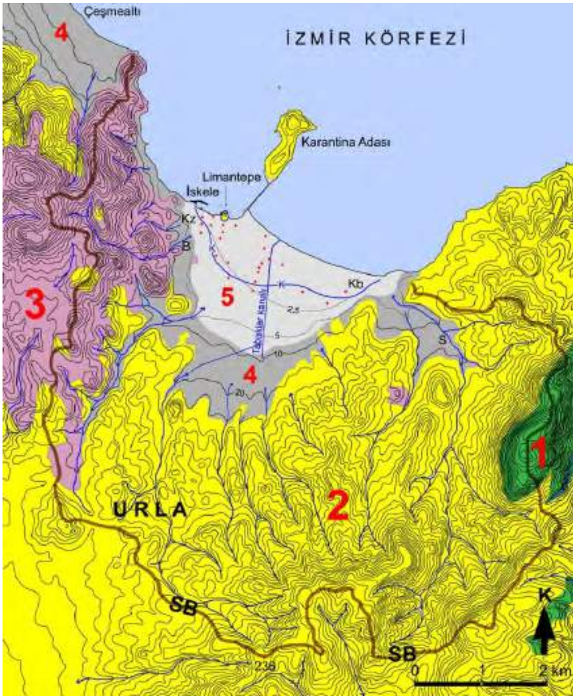
Şekil 8. Urla-Limantepe kıyı düzlüğü ve çevresinin topografya-jeoloji haritası. Topoğrafya: Eşyüksekti eğrileri 10 m aralıklarla geçirilmiştir. İskele üzlüğündeki 2,5 m eğrisi sondaj noktalarının yüzey ölçümü ve 1/25000 ölçekli haritadan enterpolasyonla çizilmiştir. SB: İskele düzlüğünün subölümü çizgisi. Litostratigrafik birimler (Kırmızı rakamlar): 5. Urla-İskele kıyı düzlüğü alüvyal örtüsü (Holosen), 4. Alüvyal-kolüvyal etek düzlüğü birikintileri, 3. Miosen (Kırıntılı ve karbonatlı gölsel birimler), 2. Miosen (Aglomera, tüfit ve asit magmatik birimler), 1. Mesozoik birimler (Kırıntılı ve karbonatlı birimler- Filiş) K: Holosen transgresyonunda denizin karaya en çok sokulduğu dönemin kıyı çizgisi (Orta Holosen: 6000 yıl kadar önce), Sondaj noktaları kırmızı ile gösterilmiştir, S: Sungurlu deresi, B: Bozavlu deresi, Kz: Klazomenai kazı alanı, Kb: Kalabak mevkii-mahallesi.
