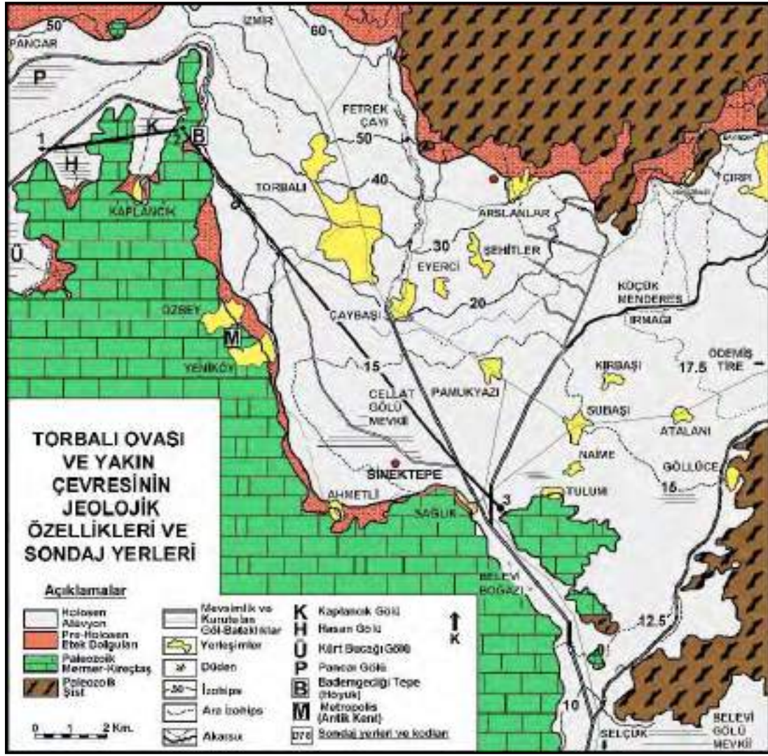
Şekil 2. Küçük Menderes ovası batı bölümünün jeolojik-topografik özellikleri (Vardar ve Sarıöz, 2006).
