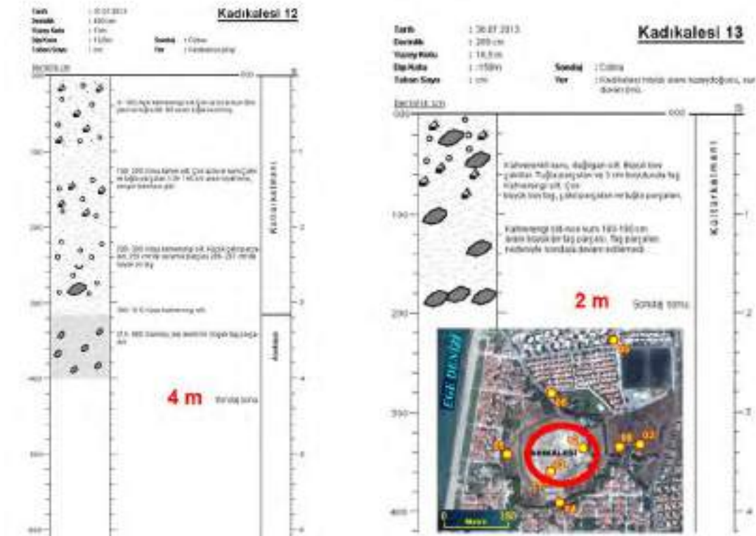
Şekil 47. Kadikalesi-12 ve 13 sondajlarına ait loglar ile sondaj yerleri.
