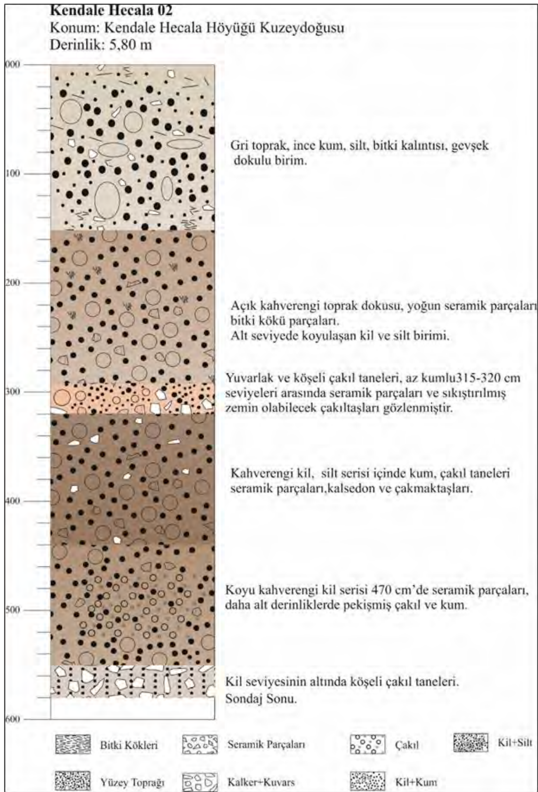
Şekil 8. Kendale Hecala 2 nolu sondaj litoloji loğu.
