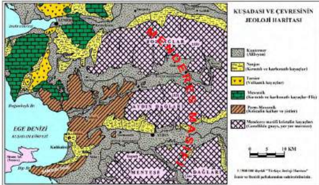
Şekil 2. Kuşadası ve çevresinin jeoloji haritası.
