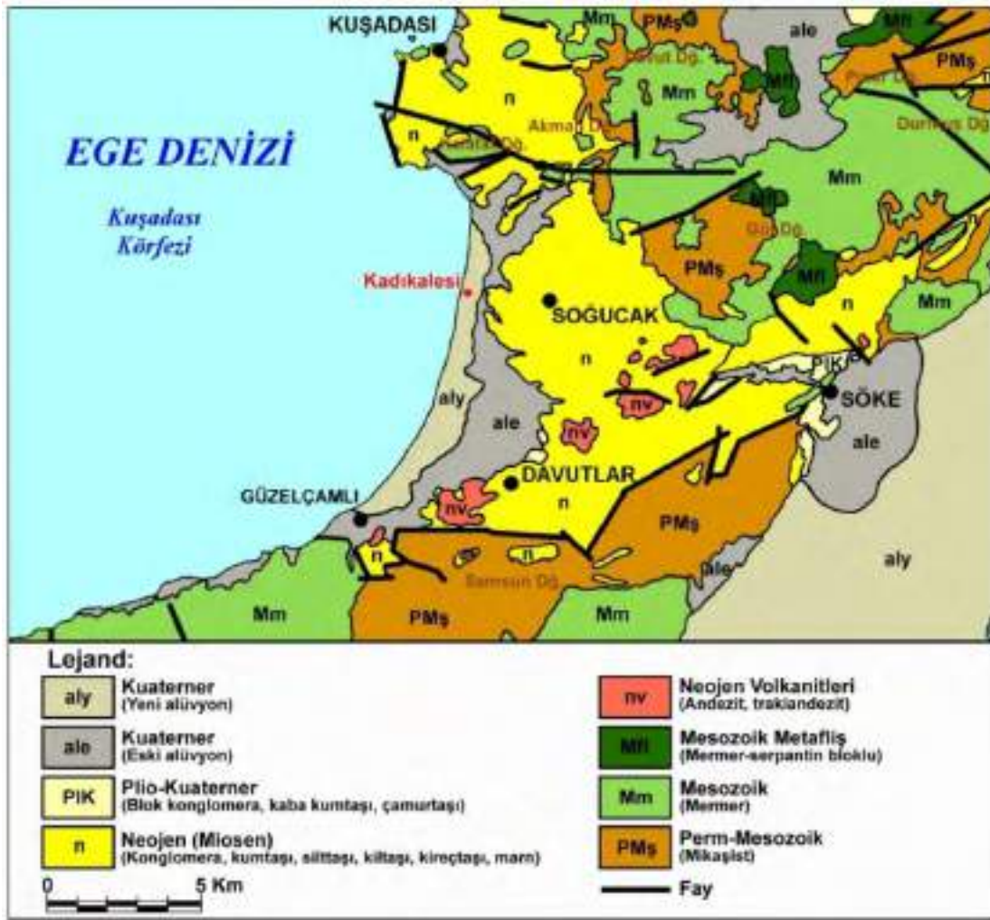
Şekil 3. Kuşadası-Davutlar kıyı düzlüğü ve çevresinin jeoloji haritası.
