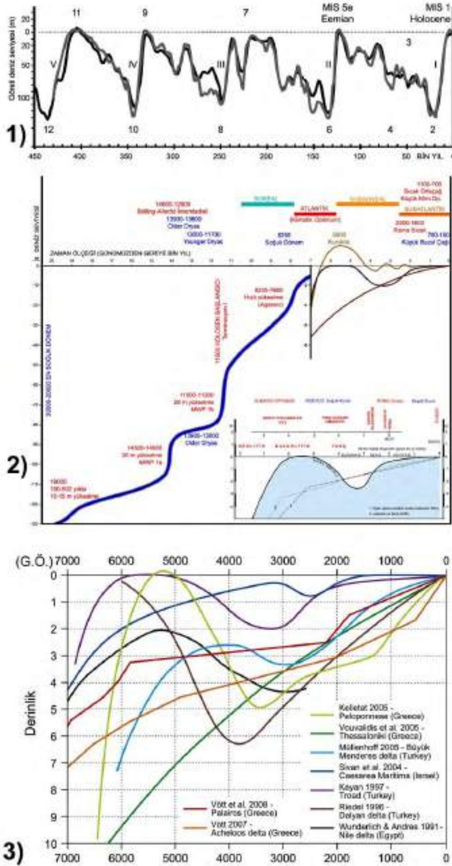
Şekil 9. Dünya denizlerinin seviye değişme eğrileri. A) Son 450 bin yılda görel deniz seviyesi değişimleri. Grafik, Kuzey Atlantik (siyah çizgi) ve Pasifik (gri çizgi) okyanuslarında birçok araştırmacı tarafından bentik organizmalarda yapılan \delta^{18}O izotop ölçümlerine dayanmaktadır (Waelbroeck vd., 2002). B) Son buzul çağı maksimumunu izleyen yaklaşık 20 bin yılda iklim ve deniz seviyesi değişimleri (Kayan, 2012). C) Son 7000 yıldaki Doğu Akdeniz (Yunanistan-Türkiye-İsrail ve Mısır) kıyılarında deniz seviyesi değişimleri (Brückner vd., 2010).
