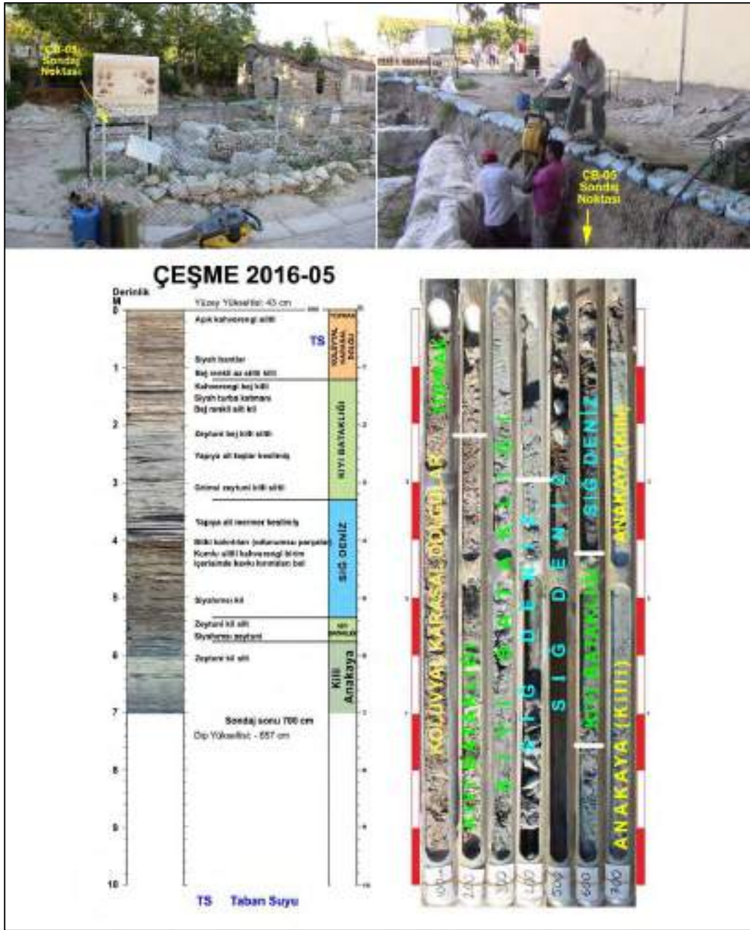
Şekil 9. ÇB-2016-05 numaralı sondaj çalışmasından görüntüler, sondaj logu-karotu ve ortam özellikleri.
