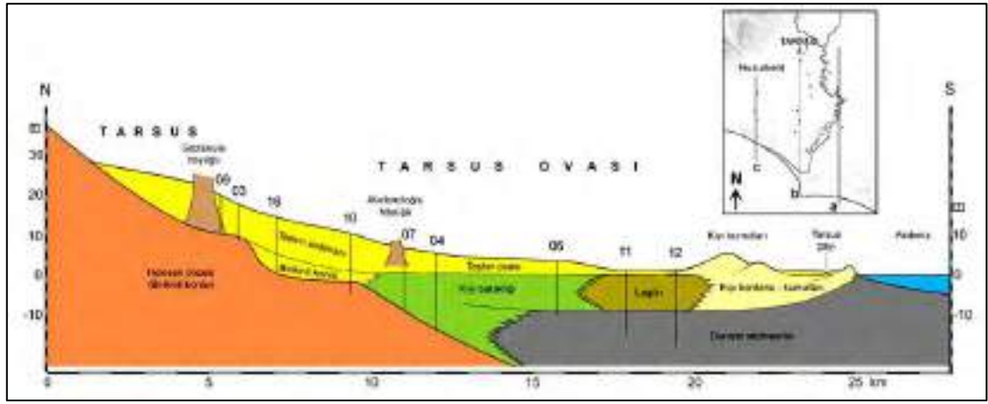
Şekil 9. Holosen öncesi birikinti konileri üzerindeki Tarsus ovasının (orta kesimi) alüvyal stratigrafisini gösteren kuzey-güney doğrultulu kesiti. Dikey çizgi ve numaraları sondajları göstermektedir. Küçük haritada “b” harfi kesit yer ve doğrultusunu gösterir.
