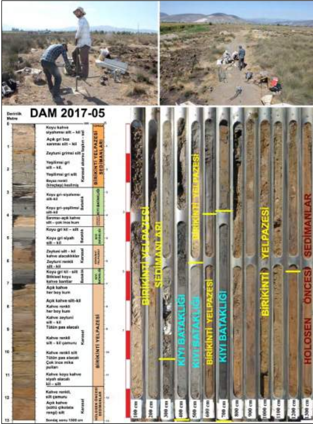
Şekil 19. Koruköy merasının batı-güneybatı köşesinde yapılan ve 13 metre derinliğe inilen DAM-2017-05 numaralı sondaj çalışmasından görüntüler, sondaj logu-karotu ve ortam özellikleri.
