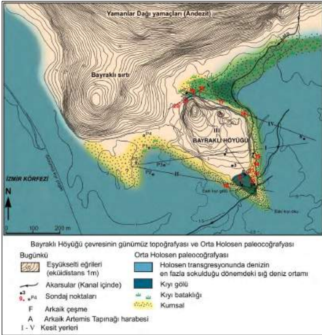
Şekil 16. Bayraklı Höyüğü çevresinin günümüz ve Orta Holosen paleocoğrafyası ile delgi sondaj yerleri. Höyüğün güney ve kuzey kesimlerdeki kıyı gölü ve bataklıklarda çökelip korunan Santorini volkanının küllerine rastlanmıştır.
