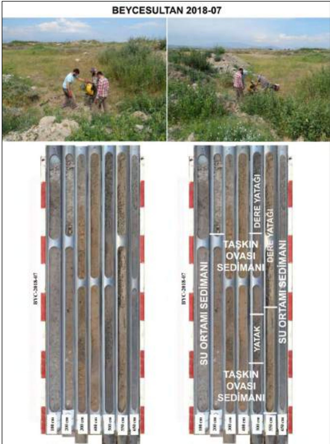
Foto 10. Beycesultan Höyüğü kuzeydoğusundaki Kanlıgöl Mevkii ortasında yapılan BYC 2018-07 numaralı delgi sondaja ait sedimanlar ve yansittıkları ortamlar.
