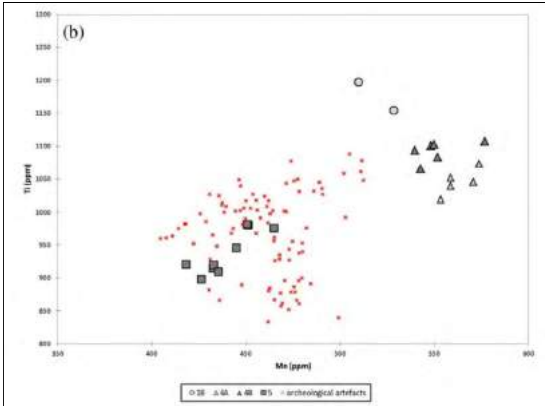
Şekil 6. Nemrut obsdiyenleri ve Yakın Doğu'daki bulunmuş 91 arkeolojik esere ait Ti-Mn ikili Diyagramı (Kaynak: Robin, 2016)
