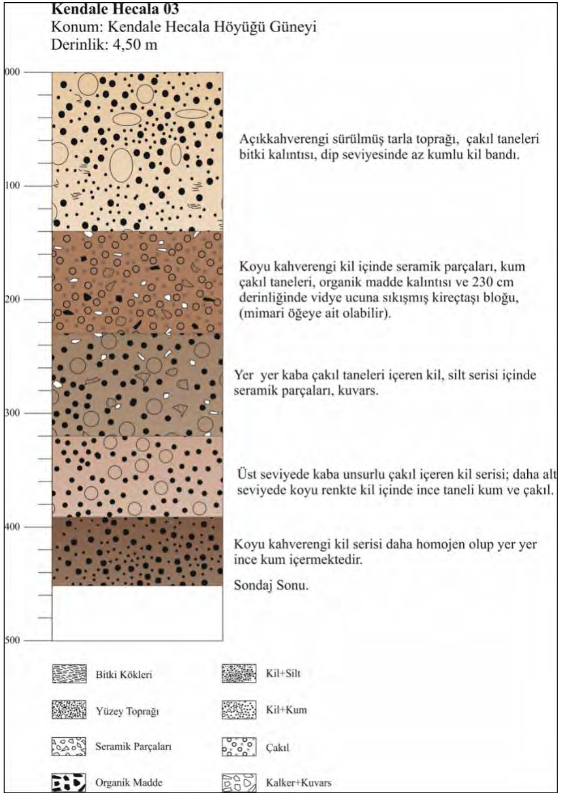
Şekil 9. Kendale Hecala 3 nolu sondaj litoloji logu
