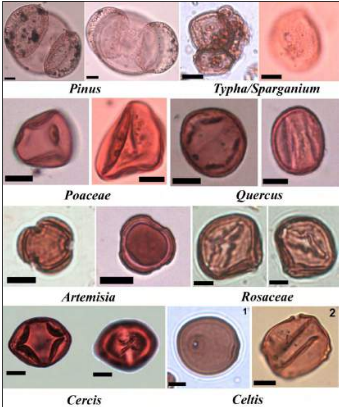
Şekil 8. Bornova 03 numaralı sondaja ait Palinomorflar (Polenler).
