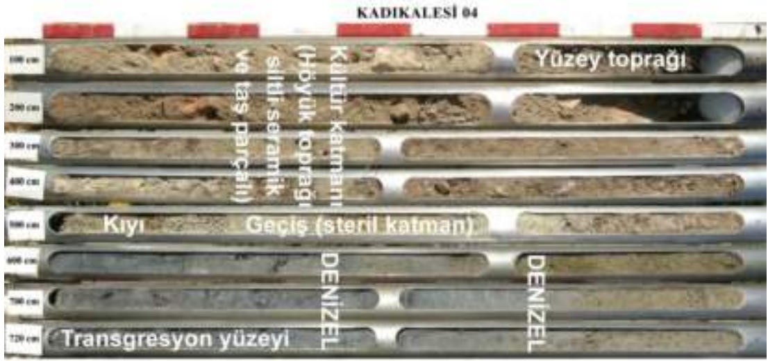
Şekil 28. Kadikalesi-04 sondajına ait sedimanların ortam özellikleri.
