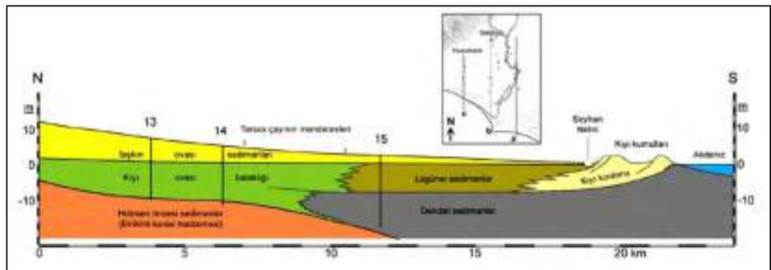
Şekil 11. Holosen öncesi birikinti konileri üzerindeki Tarsus ovasının (doğu kesimi) alüvyal stratigrafisini gösteren kuzey-güney doğrultulu kesiti. Dikey çizgi ve numaraları sondajları göstermektedir. Küçük haritada “a” harfi kesit yer ve doğrultusunu gösterir.
