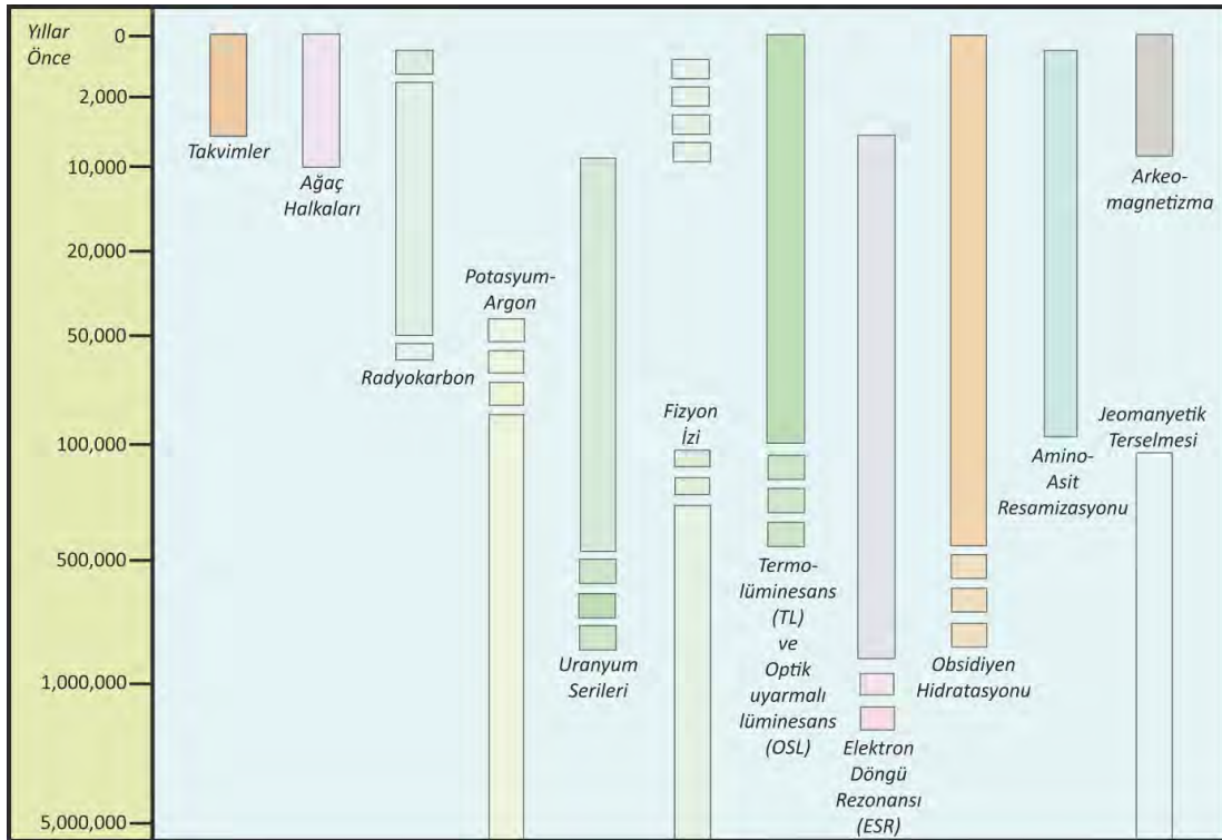
Şekil 1. Jeoarkeoloji çalışmalarında kullanılan tarihlendirme yöntemleri.
