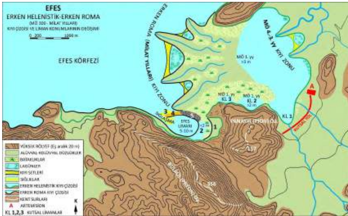
Şekil 12. Efes ve Artemision çevresinin Helenistik dönemdeki (M.Ö. 300-1) paleocoğrafya haritası. Gemilerin muhtemel erişimini belirtmek amacıyla bazı noktalarda deniz suyu derinlikleri gösterilmiştir (mavi). Küçük Menderes deltası sürekli olarak denize doğru ilerledikçe Artemision'daki Kutsal Limanın yavaş yavaş batıya doğru yerinin değiştirilmesi gerekmiştir (KL 1, 2, 3). Bülbül ve Panayır dağlarının kavşağındaki Lysimachus'un "Arsinoeia" kentinin (1) kıyısı delta önü siltleri ve yapı enkazı ile hızla dolmuştur (2). Helenistik Çağda Attalus II Philadelphus'un liman ağzındaki çalışmaları hipotetik bir değerlendirme olarak gösterilmiştir. Ancak orta Helenistik mühendislerinin çalıştığı liman, aşağı kentin üzerine inşa edildiği geç Helenistik / en erken Roma İmparatorluk dolgusunun (2) altında doğuya doğru uzanıyor olabilir. (3) Limandaki silt sıklıkları, (4) yapısıyla liman girişini daraltan set-mendirek ve (5) Roma döneminde yerleşme alanı olan, liman kuzeyindeki büyük set-mendirek.
