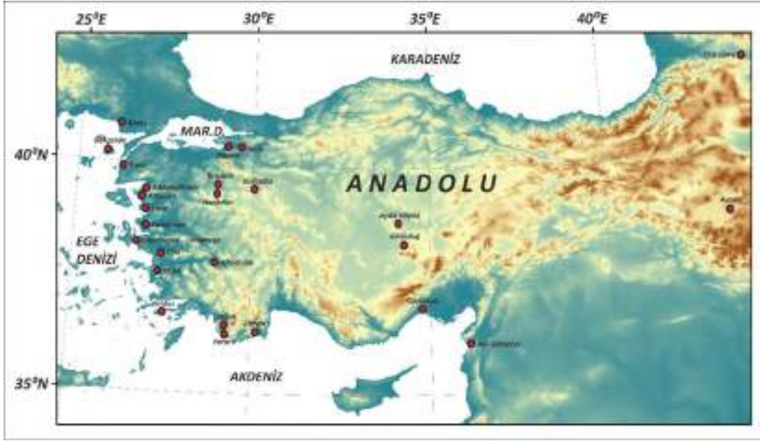
Şekil 2. Anadolu’da farklı bölgelerde delgi-sondajlar kullanılarak yapılan jeoarkeoloji çalışmaları.
