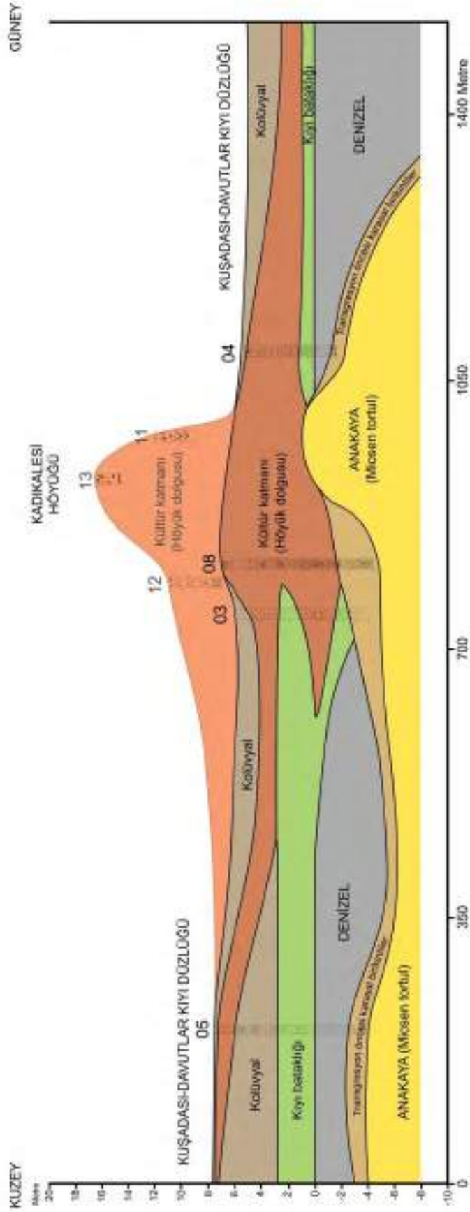
Şekil 49. Kadikalesi höyüğü ve çevresinde yapılan delgi sondaj sonuçlarına göre hazırlanan Kuzey-Güney doğrultulu Doğu taraf kesiti (Numaralar sondaj yerlerini göstermektedir) (Not: Gerideki 12, 13 ve 11 numaralı sondajların bulunduğu silik höyük görüntüsü batı bölümden korelasyonla aktarılmış olup Kadikalesi höyüğünün bütününe yansıtılmak için kesite eklenmiştir)
