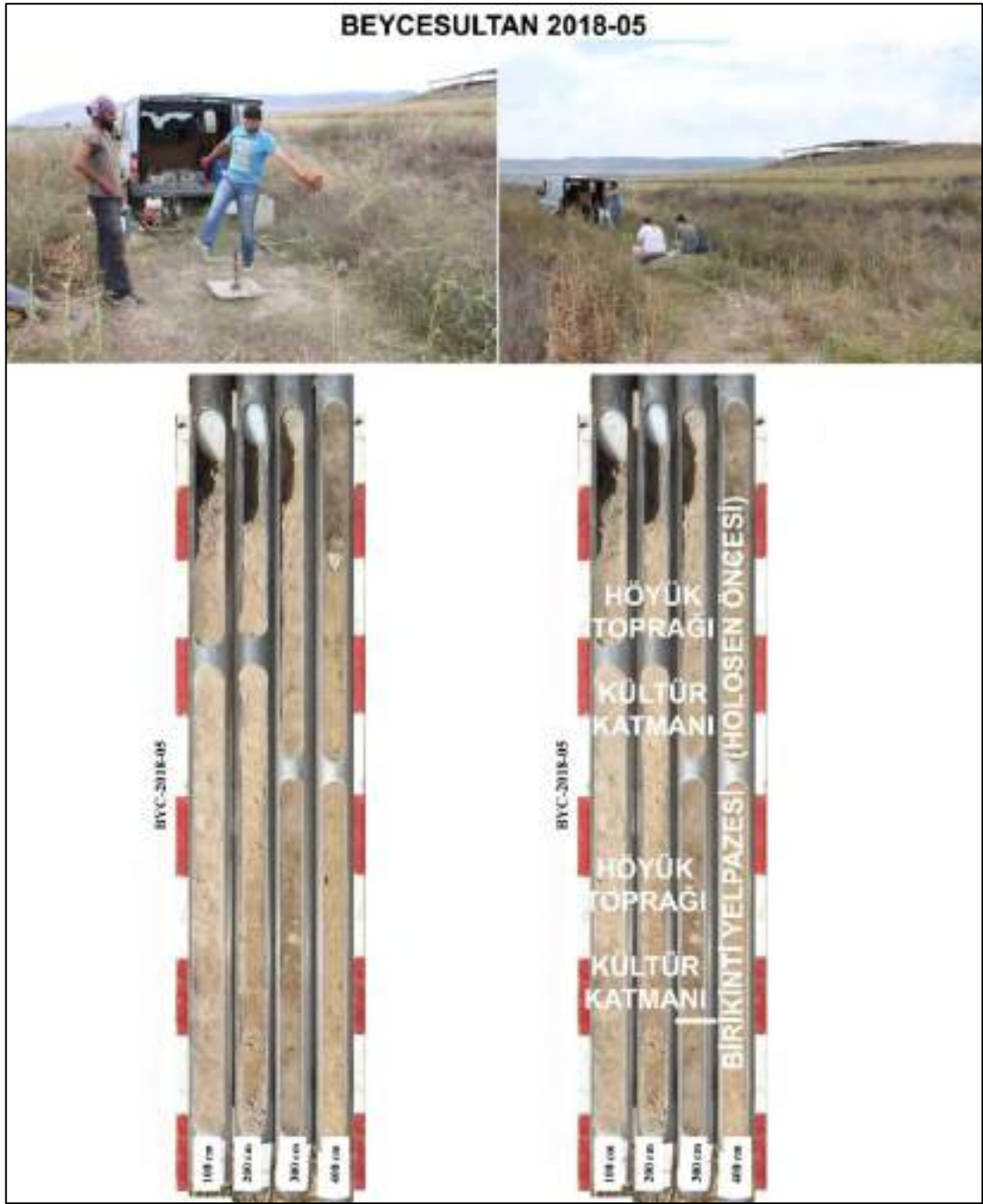
Foto 8. Beycesultan Höyüğü güney eteğinde yapılan BYC 2018-05 numaralı delgi sondaja ait sedimanlar ve yansıttıkları ortamlar.
