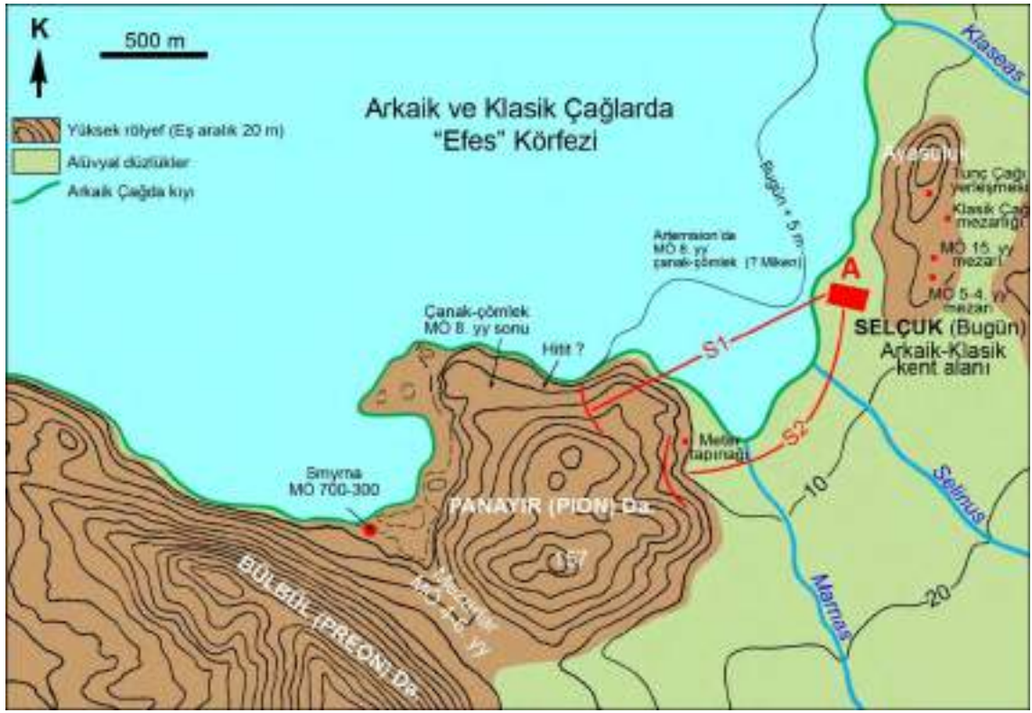
Şekil 6. Arkaik ve Klasik çağlarda, Selçuk (Ayasuluk) tepesi ile Panayır (Pion) dağı arasında, Artemision yakınındaki deniz girintisinin kıyılarını gösteren paleocoğrafya haritası. Büyük Artemision tapınağı ve onun altındaki daha eski tapınaklar, eski Derbent (Selinus) deresinin alüvyon yelpazesinden Efes körfezine doğru uzanan küçük bir çıkıntının üzerinde yapılmıştı. Herodot (M.Ö. 5. yüzyıl), İyonyalı Yunanistan göçmen yerleşiminin Artemision'dan 7 stadia (yaklaşık 1300 m) uzaklıkta olduğunu belirtir. Haritadaki S1 çizgisi Artemision'dan kuş uçuşu 7 stadia uzaklığı göstermektedir. S2 çizgisi ise kutsal liman çevresindeki kıyı yüründüğünde 7 stadia uzaklıktaki mesafede çizilecek yayı göstermektedir. Buna göre, ~ M.Ö. 1000 yıllarında, Androclus'un henüz bulunamamış olan İyon-Yunan yerleşme yerinin güneyde "Yedi Uyuyanlar Mağarası" yakınında, Panayır (Pion) dağı güneydoğu yamacında veya eski Marnas (veya Selinus) deresi kenarındaki alüvyal düzlükte bir yerde olacağını varsayıyoruz. Kıyı çizgisinin belirlenmesinde İ. Kayan'ın Şekil 2'de gösterilen, yayımlanmamış delgi sondaj noktalarından yararlanılmıştır.
