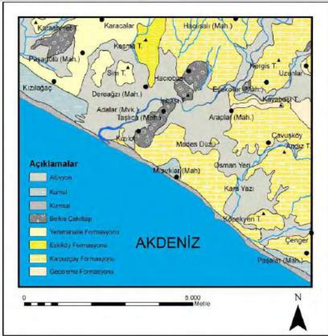
Sekil 3. Araştırma alanının jeoloji haritası (Akay ve Uysal 1985'ten alınmıştır).
