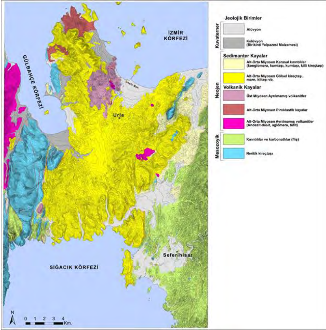
Şekil 7. Urla Yarımadası ve çevresinin jeoloji haritası.
