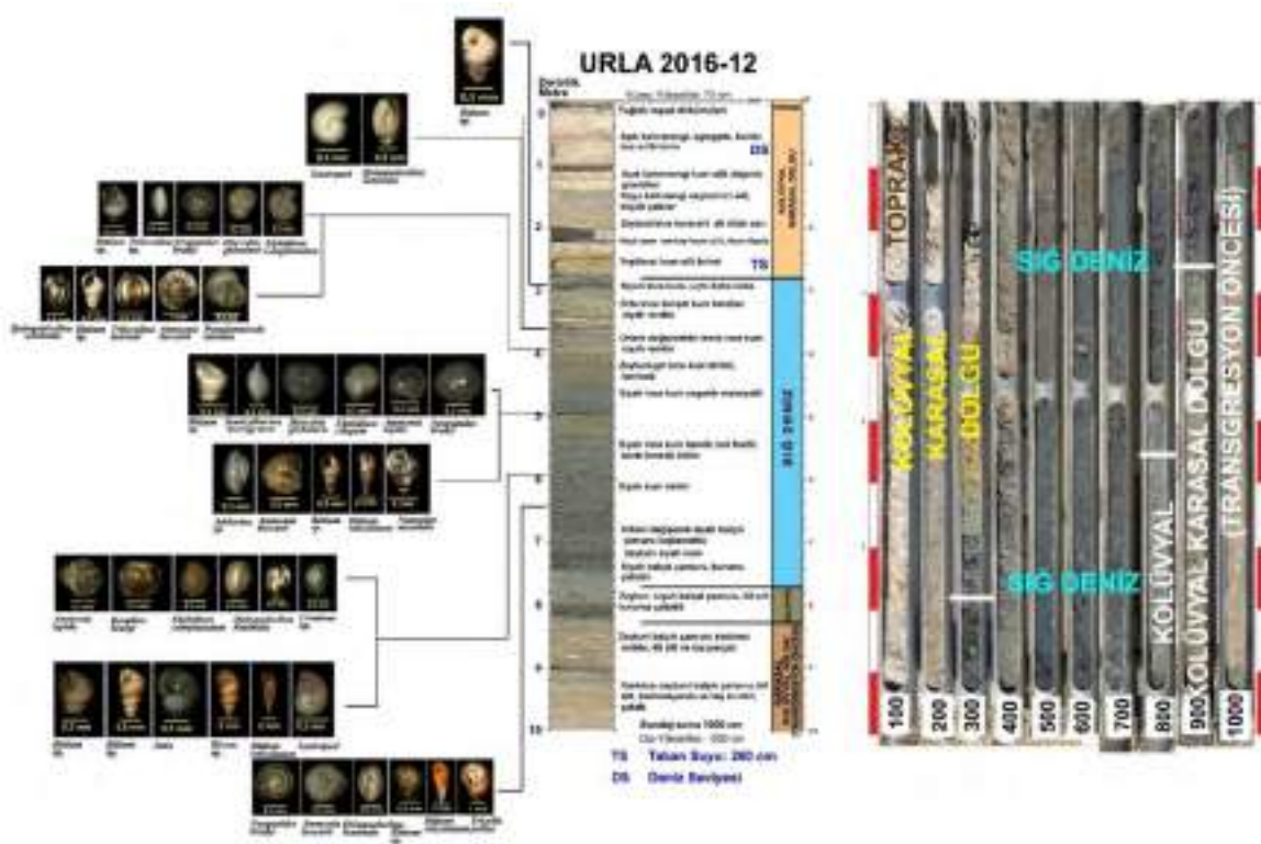
Şekil 25. Urla 2016-12 (15) numaralı sondaja ait log, sedimanların birikme ortamları ve fosillerin seviyelerine göre dağılımı.
