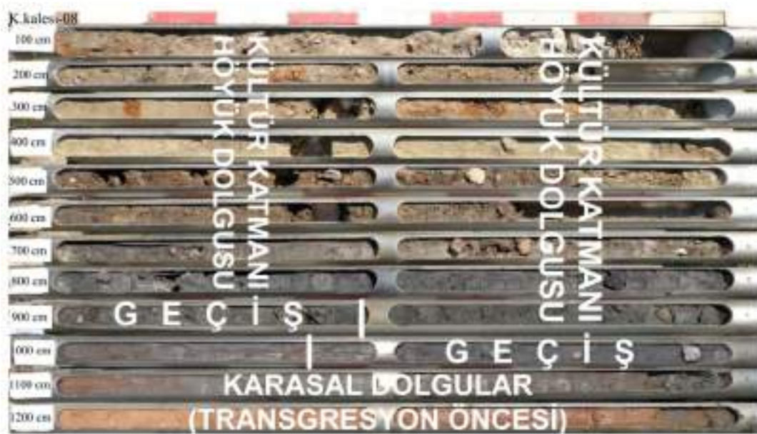
Şekil 45. Kadıkalesi-08 sondajına ait sedimanların ortam özellikleri.
