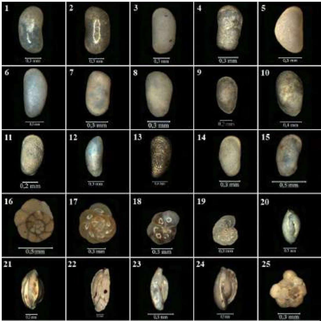
Levha 1. Sariçay Ovasında yapılan delgi sondajlarda rastlanan baskın fosiller: Ostracodlar ve Foraminiferler. 1. Candona sp.; 2. Candona parallela pannonica ; 3. Pseudocandona sp.; 4. Ilyocypris gibba ; 5. Heterocypris salina ; 6. Cyprideis sp.; 7. Bacuniella sp.; 8. Loxoconcha sp.; 9. Loxoconcha sp.; 10. Loxoconcha elliptica ; 11. Leptocythere sp.; 12. Argilloecia sp.; 13. Cytheridea neapolitana ; 14. Leptocythere sp.; 15. Leptocythere bituberculata ; 16. Ammonia sp.; 17. Ammonia tepida ; 18. Nonion sp.; 19. Nonion depressulum ; 20. Quinqueloculina seminula ; 21. Adelosina sp.; 22. Adelosina sp.; 23. Adelosina mediterraneensis ; 24. Triloculina marioni ; 25. Planorbulina mediterraneensis .
