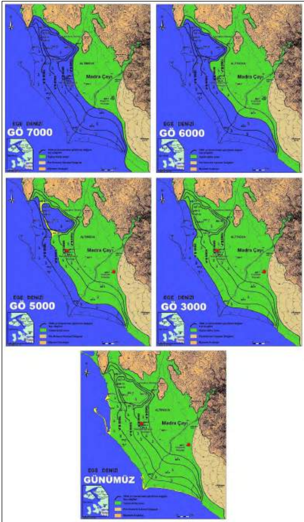
Şekil 1. Madra Çayı Deltası'nın (Altınova) Holosen kıyı değişimleri (Vardar, 2010).
