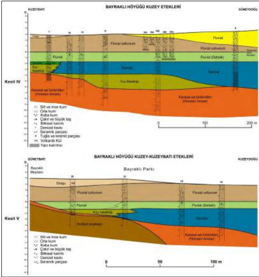
Şekil 18. Bayraklı Höyüğü sondaj sonuçlarına göre hazırlanan kuzeybatı-güneydoğu (IV) ve güneybatı-kuzeydoğu doğrultulu (V) kesitler. Kesit yerleri için Şekil 16'ya bakınız.
