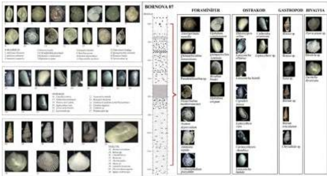
Şekil 7. Bornova sondajlarından alınan sedimanlar içindeki makro ve mikro fosillerin analizleri yapılarak ortam belirleme açısından yararlanılmıştır. Bütün sondajlarda gözlenen baskın foraminifer, ostrakod ve molusk türleri (solda) ile Bornova 07 numaralı sondajın sedimanlarındaki mikro ve makrofosiller (sağda).
