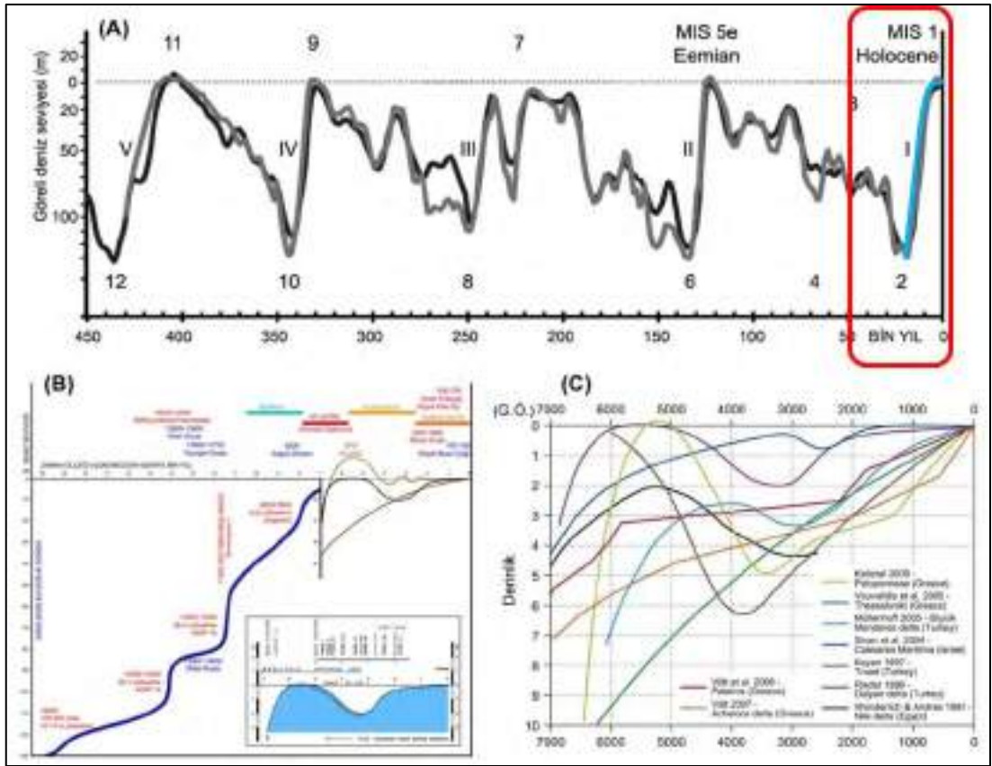
Şekil 10. Dünya denizlerinin seviye değişme eğrileri. A) Son 450 bin yılda görelî deniz seviyesi değişimleri. Grafik, Kuzey Atlantik (siyah çizgi) ve Pasifik (gri çizgi) okyanuslarında birçok araştırmacı tarafından bentik organizmalarda yapılan \delta^{18}O izotop ölçümlerine dayanmaktadır (Waelbroeck ve ark., 2002). B) Son buzul çağı maksimumunu izleyen yaklaşık 20 bin yılda iklim ve deniz seviyesi değişimleri (Kayan, 2012). C) Son 7000 yıldaki Doğu Akdeniz (Yunanistan- Türkiye-İsrail ve Mısır) kıyılarında deniz seviyesi değişimleri (Brückner vd., 2010).
