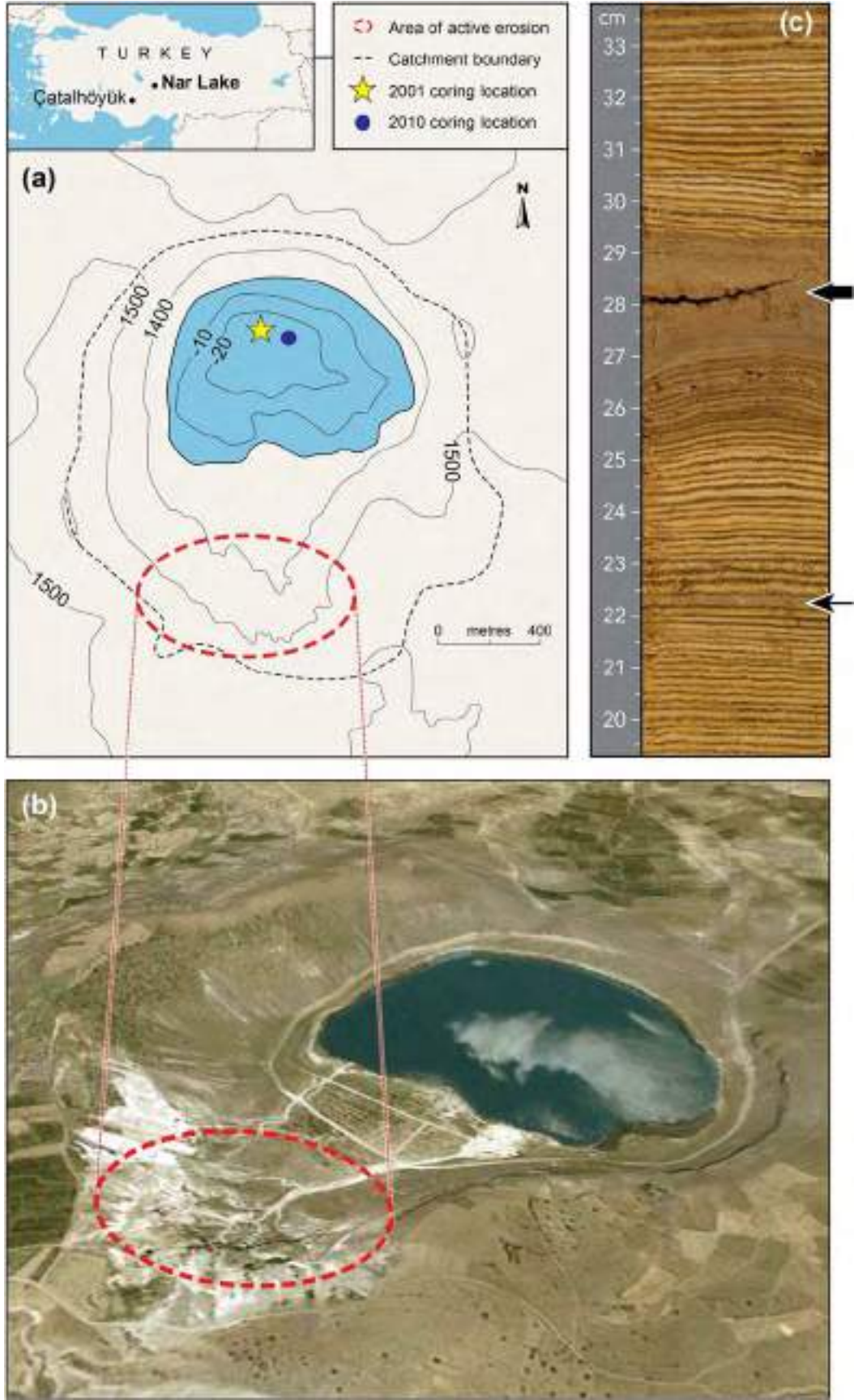
Şekil 1. (a) Nar Gölü ve havzasındaki sondaj noktaları ve badlands alanını gösteren konum haritası; (b) göl ve havzasının oblik uydu görüntüsü (Google Earth); (c) 1. Birimi gösteren karot kesiti, biri kalın, diğeri ince olan kırıntılı sedimanlarla (okla gösterilen) kesintiye uğrayan varırlar görülmektedir.
