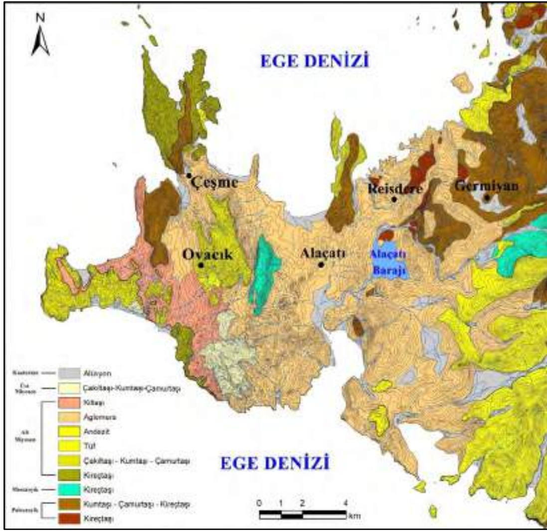
Şekil 3. Çeşme Bağlararası ve yakın çevresinin jeolojik özellikleri (MTA 1/100000 ölçekli jeoloji haritasından yararlanılarak hazırlanmıştır).
