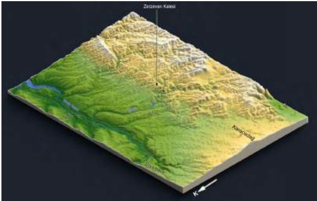
Şekil 2. Zerzevan Kalesi'nin konumunu gösteren 3 boyutlu sayısal arazi modeli.
