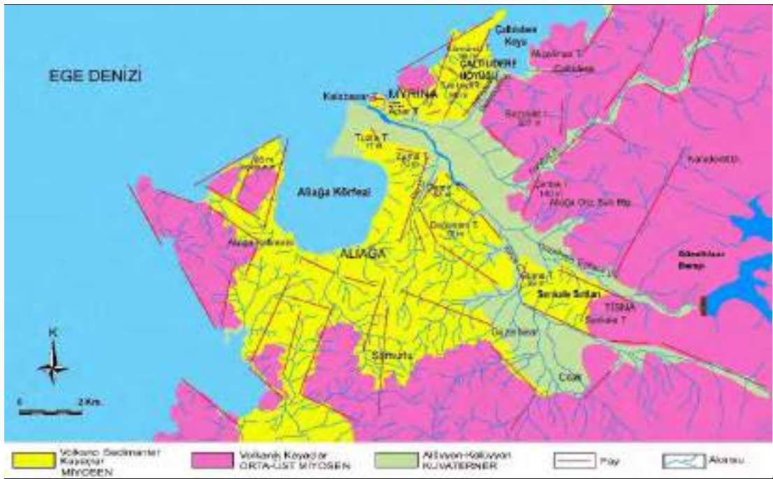
Şekil 3. Myrina ve Aliaga çevresinin ana jeolojik birimleri ve tektoniği (Vardar, 2017).
