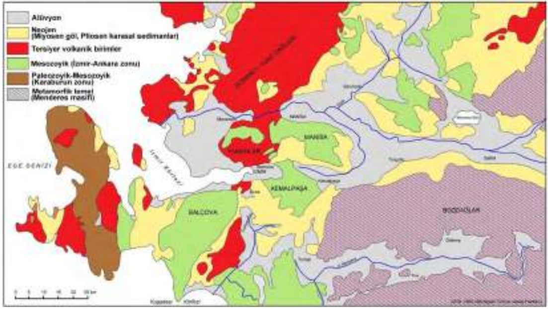
Şekil 9. Bornova Ovası ve Bayraklı Höyüğü çevresinin jeoloji haritası.
