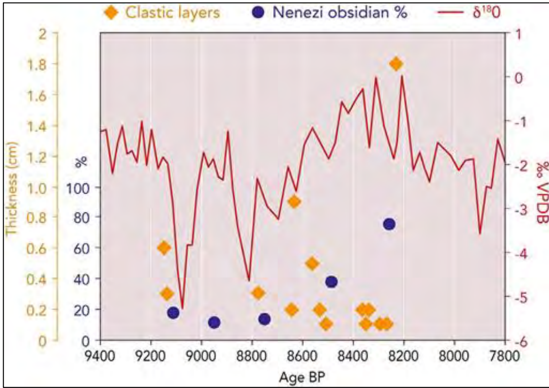
Şekil 5. NAR 10 karotuna göre Çatalhöyük'te bulunan Nenezi obsidiyenlerinin oranı (sol ekseninde % olarak gösterilmektedir, Carter 2011) ile Neolitik'teki erozyonda ve iklimdeki değişimler (sol taraftaki ekseninde klastik tabaka kalınlıkları cm olarak verilmiştir, sağdaki ekseninde ise O^{18} izotop analizine göre iklim değişimleri gösterilmiştir) (BP: Günümüzden Önce).
