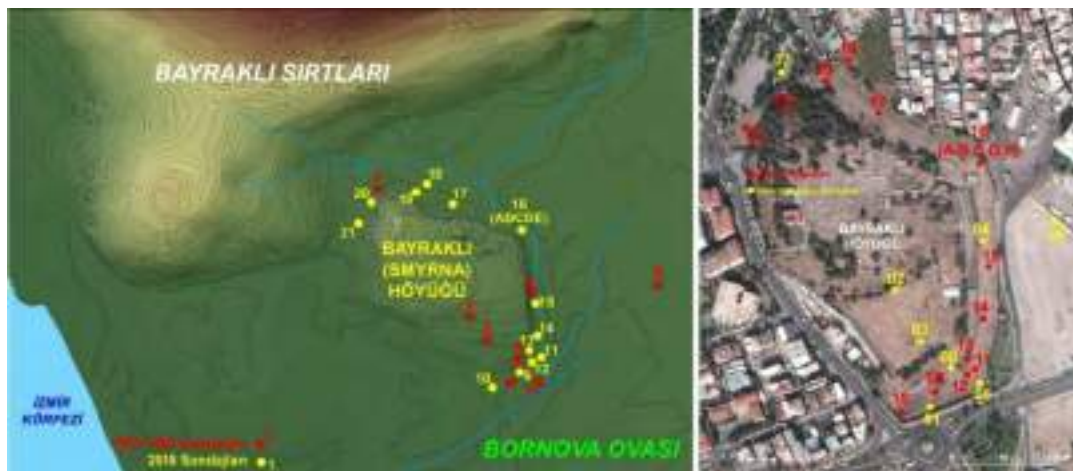
Şekil 4. Bayraklı sırtları ile Höyüğünün hipsometrik haritası (solda) ve uydu görüntüsü (sağda) üzerinde delgi sondaj yerleri.
