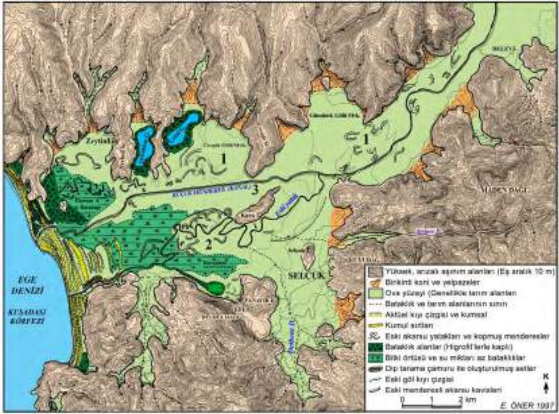
Şekil 1. Küçük Menderes (antik Cayster-Kaystros) ırmağı taşkın ovasında, yatay ve dikey yöndeki sedimentasyon süreçleri ile oluşan jeomorfolojik birimler: (1) Terk edilmiş, eski menderes halkalarının kalıntıları, (2) daha yeni, 20. yüzyıl başlarına ait terk edilmiş yatak kalıntıları, (3) güncel drenaj ve sulama kanalı. Ertuğ Öner tarafından, hava fotoğrafları ve uydu görüntülerinden çizilmiştir (Öner 1997).
