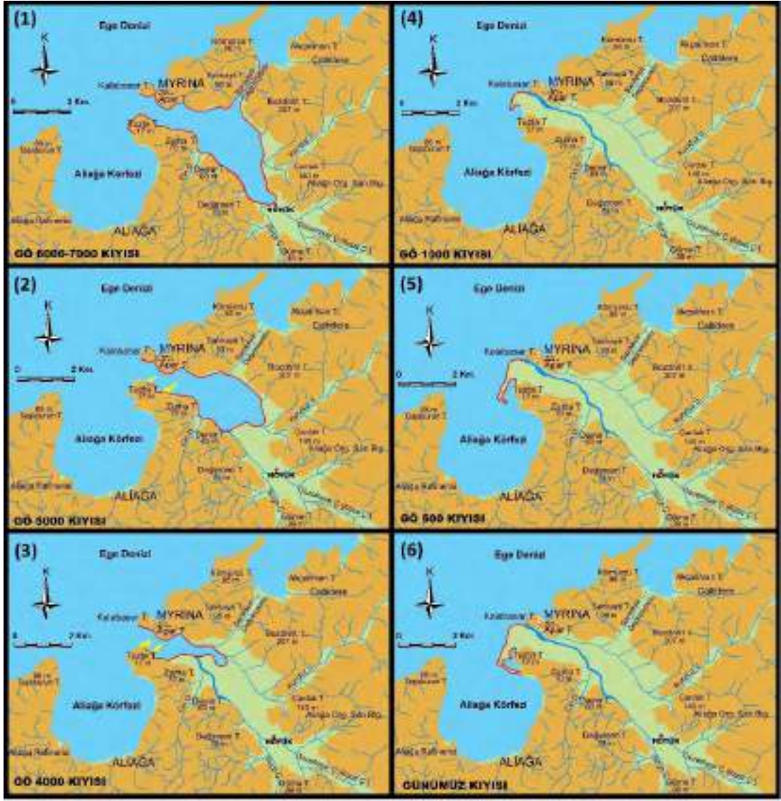
Şekil 11. Güzelhisar kıyı ovasının paleocoğrafyası ve eski kıyı çizgileri.
