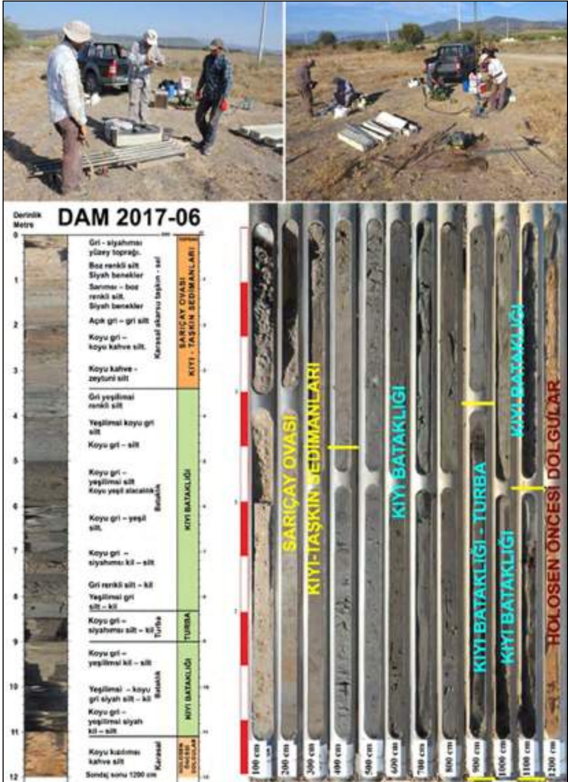
Şekil 20. Koruköy merasının batı-kuzeybatı köşesinde yapılan ve 12 metre derinliğe inilen DAM-2017-06 numaralı sondaj çalışmasından görüntüler, sondaj logu-karotu ve ortam özellikleri.
