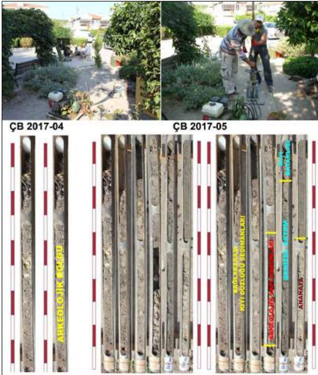
Şekil 19. ÇB-2017-04 ve ÇB-2017-05 numaralı sondaj çalışmalarından görüntüler, sondaj logu ve ortam özellikleri.
