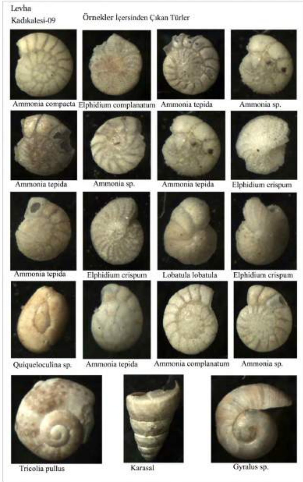
Şekil 37. Kadıkalesi-09 sondajında görülen Foraminifer, Ostrakod ve Gastropod cins ve türlerine ait levha.
