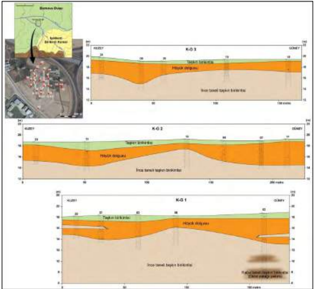
Şekil 15. Yeşilova Höyüğü kuzey-güney doğrultulu kesitleri.
