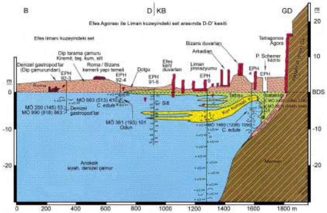
Şekil 9. Bülbul (Preon) dağı ile Panayır (Pion) dağı arasındaki çukurluk tabanında P. Scherrer'in Tetragonos Agora kazılarında, Roma'nın Efes kentini katederek batıya uzanan jeolojik kesit. Kent, Küçük Menderes'in biriktirdiği denizel silt, kıyı sedimanları ve bataklıkların üzeri yıkıntı atıklarıyla doldurularak kazanılan alanda inşa edilmiştir. Kesitin batı kesimi, limanın kuzeyinde dip taraması ve yıkıntı atıklarıyla oluşturulan büyük setin üzerinde uzanmaktadır.
