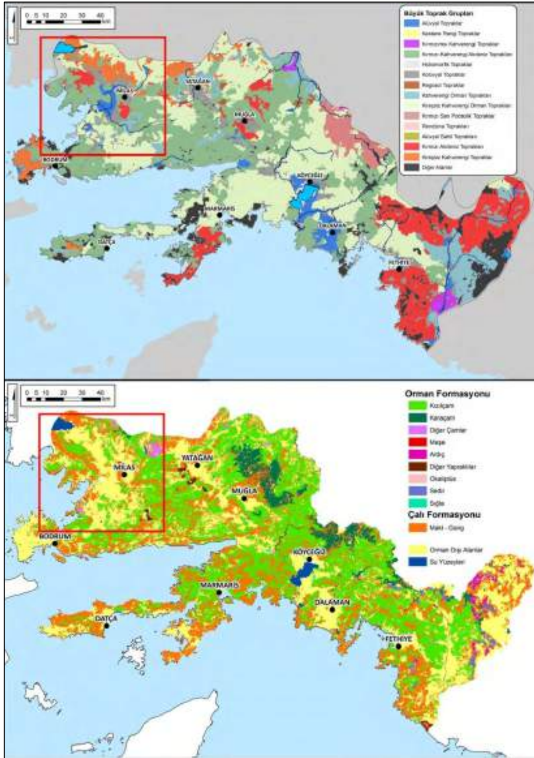
Şekil 4. Çalışma alanı ve çevresinin büyük toprak grupları (üstte) ve bitki örtüsü haritası (altta) (Yavaşlı, 2015'ten alınmıştır).
